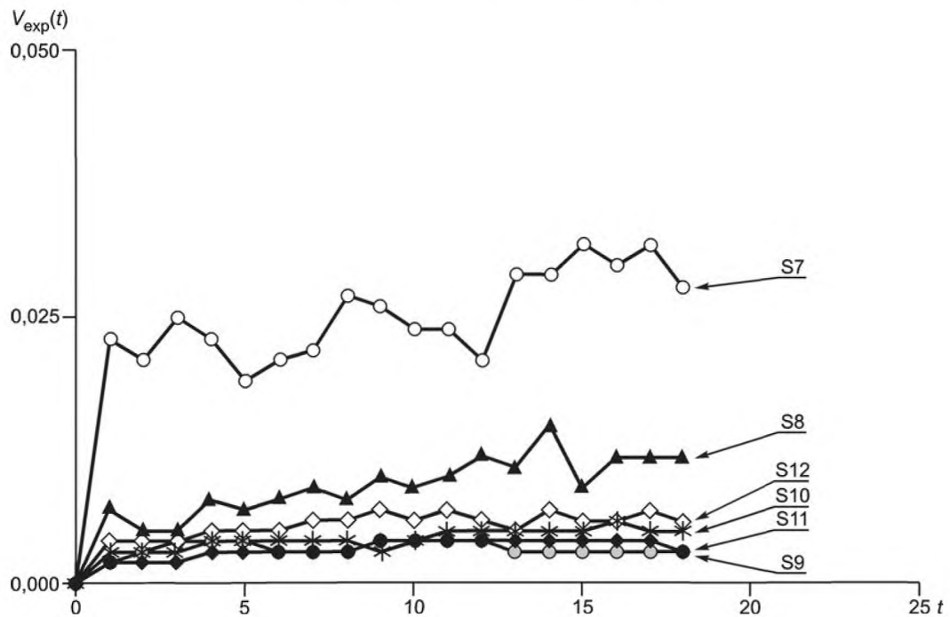
Рисунок С. 16 — Вариограмма для S7 — S12
