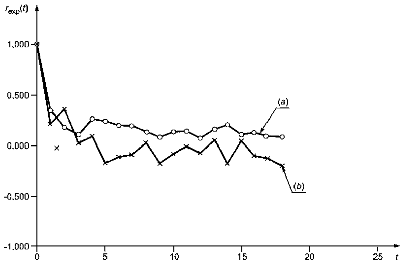
Рисунок С.5 — Коррелограммы для w_{Si}(a) и w_{Si}(b)
