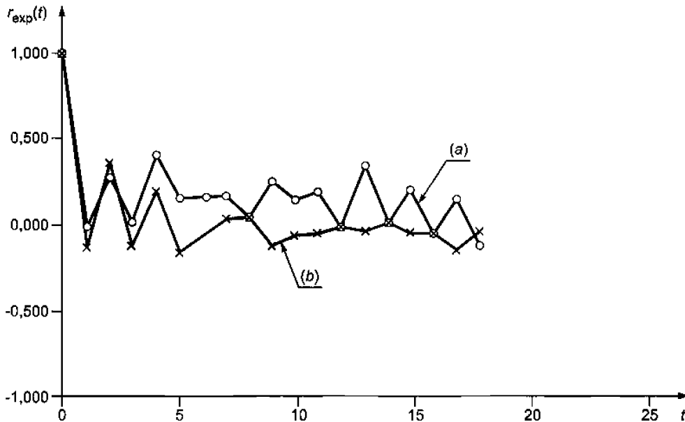
Рисунок С.7 — Коррелограммы для w_{Su}(a) и w_{Su}(b)
