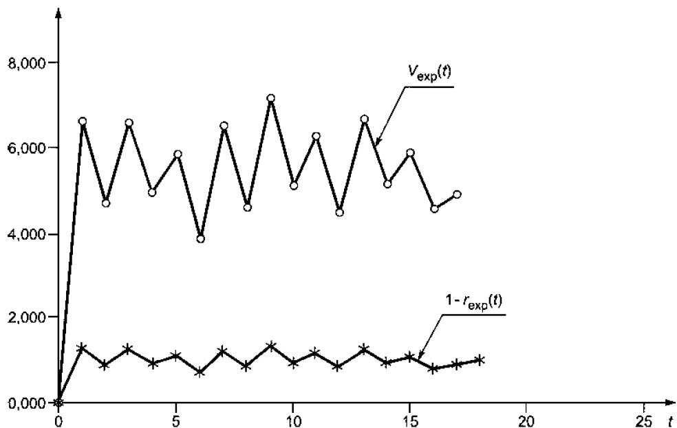
Рисунок С.8 — Соотношение между V_{exp}(t) и [1 - r_{exp}(t)] для P_{mi}(a)
