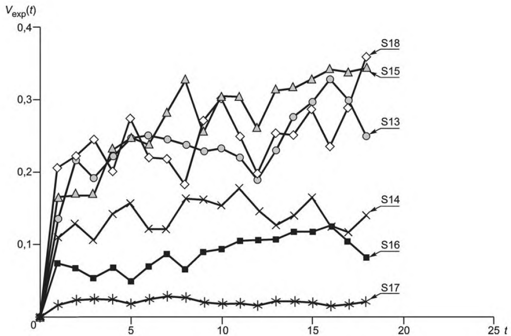
Рисунок С. 17 — Вариограмма для S13—S18
