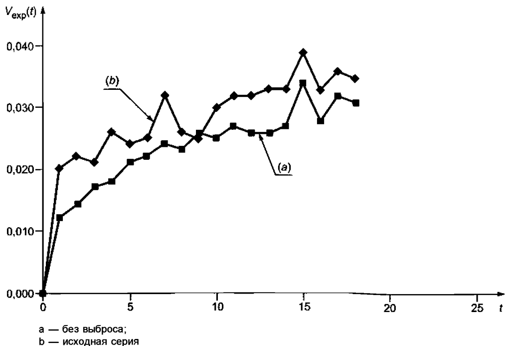
Рисунок С.14 — Вариограмма для серии №1
