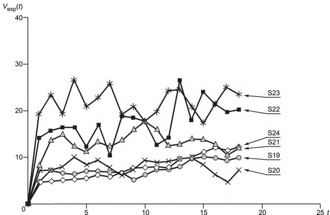
Рисунок С.19 — Вариограмма распределения частиц для S19 — S24
