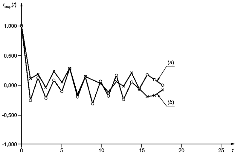
Рисунок С.3 — Коррелограммы P_m(a) и P_m(b)
