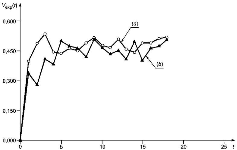
Рисунок С.4 — Вариограммы для w_S(a) и w_S(b)
