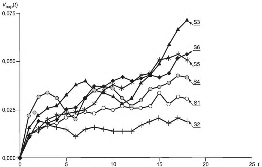
Рисунок С. 15 — Вариограмма для S1 — S6
