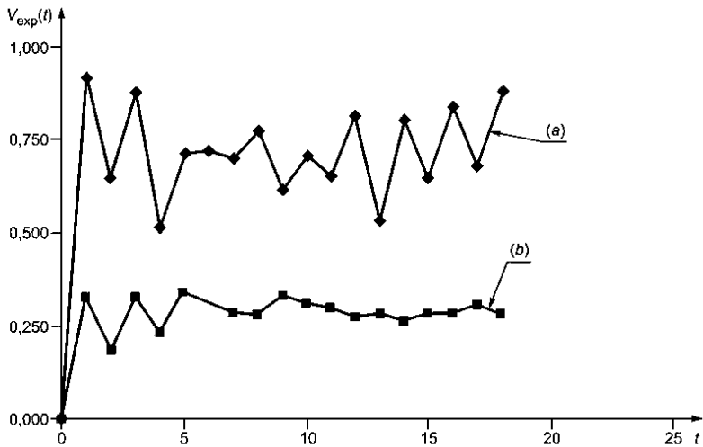
Рисунок С.6 — Вариограммы для w_{Su}(a) и w_{Su}(b)
