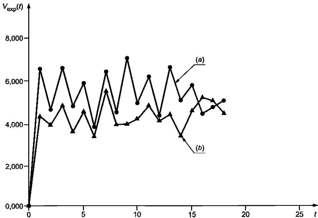
Рисунок С.2 — Вариограммы P_{mi}(a) и P_{mi}(b)
