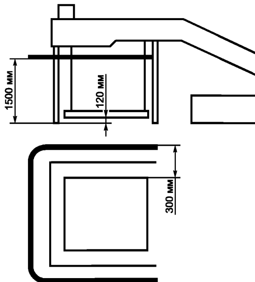
Рисунок 7 — Защита отклоняющимися частями станины машины
