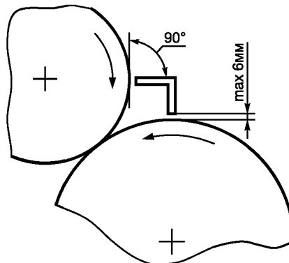
Рисунок 3 — Защита места затягивания с помощью неподвижной планки
