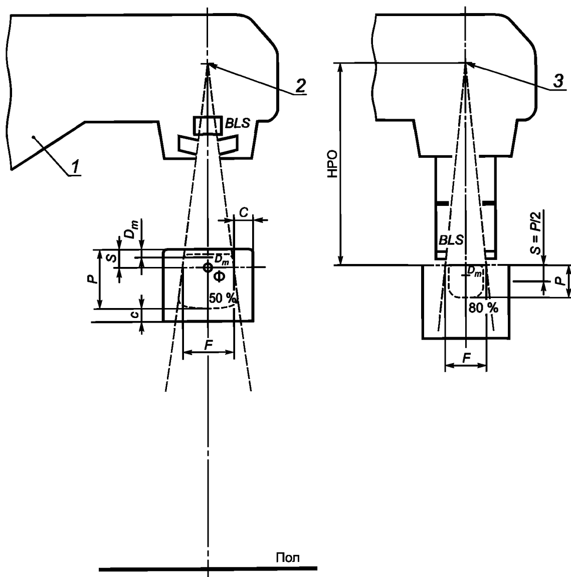
1 — ШТАТИВ; 2 — виртуальный источник ТОРМОЗНОГО ИЗЛУЧЕНИЯ; 3 — виртуальный источник ЭЛЕКТРОННОГО ИЗЛУЧЕНИЯ; \Phi — ИЗОЦЕНТР; S — стандартная измерительная глубина; P — величина, характеризующая качество проникающего ИЗЛУЧЕНИЯ; c — часть ФАНТОМА, внутри примыкающая к его граничным плоскостям; D_m — максимальное значение глубины дозы на ОСИ ПУЧКА ИЗЛУЧЕНИЯ; BLS — система коллимирования ПУЧКА ИЗЛУЧЕНИЯ; F — размер ПОЛЯ ОБЛУЧЕНИЯ; HPO — нормальное расстояние ОБЛУЧЕНИЯ
