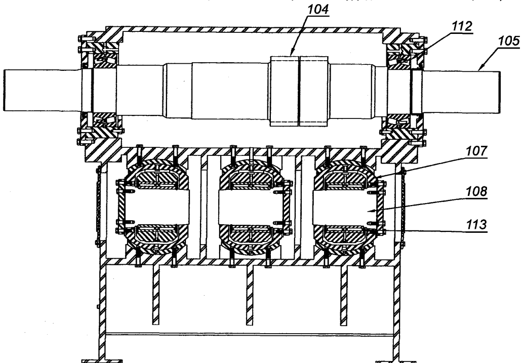
Рисунок В.3 — Поперечное сечение через вал-шестерню и кресткопф (номенклатуру деталей см. в таблице В.1)
