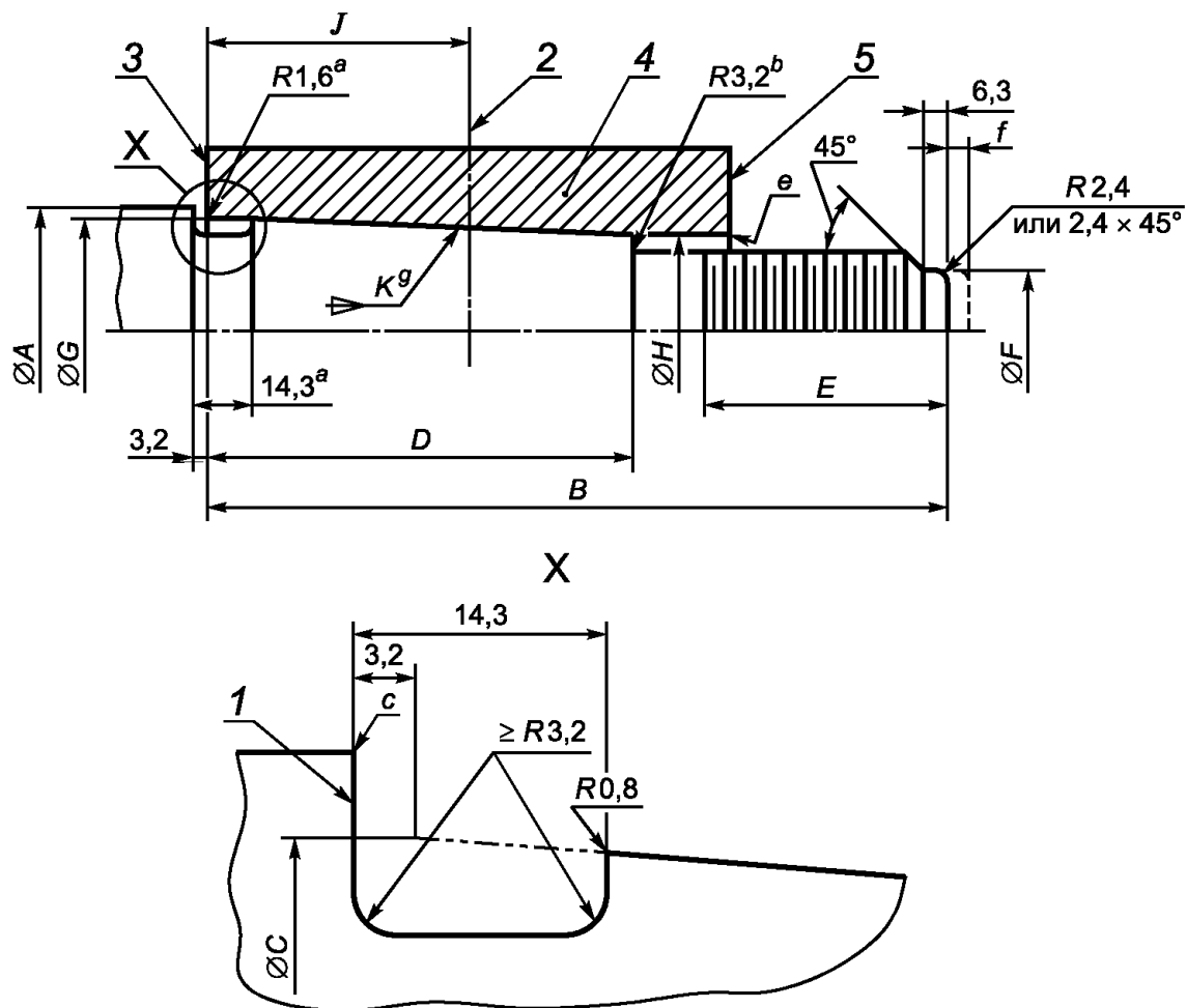
1 — заплечик штока M ; 2 — геометрическая ось поршня (в сборе); 3 — заплечик N , заплечик поршня, штоковая полость: а — максимальный размер; b — минимальный размер; с — фаска \leq 0,5 мм; j — длина до центральной оси поршня; B — длина штоковой полости; X — галтель и диаметр выточки, нагартованной при холодной обработке 4 — поршень; 5 — заплечик P , заплечик поршня, конец резьбы: e — фаска; f — максимальное удлинение хвостовика 3,2 мм; g — конус; R — радиус или фаска
