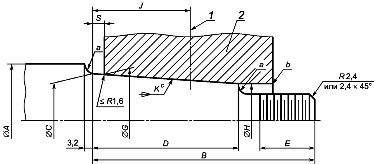
1 — центровая линия поршня (положение после крепления); 2 — поршень; а — галтель, радиус галтели R = 3 мм на каждом выступе поршня; b — фаска; с — конусность
