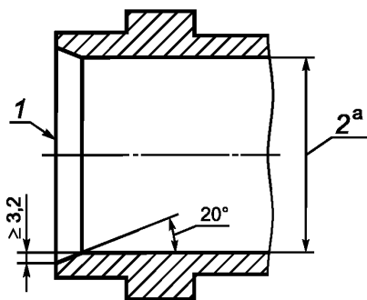
1 — входной торец плунжера; 2 — отверстие втулки; а — допуск номинального диаметра: \begin{matrix} +0,13 \\ 0 \end{matrix} мм
