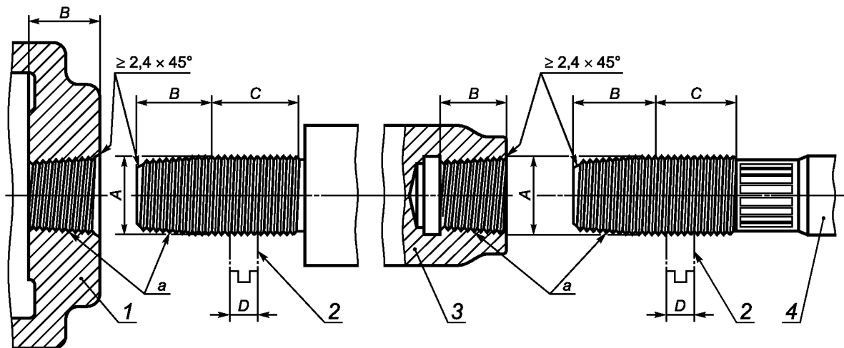
1 — ползун; 2 — контргайка; 3 — удлинение ползуна; 4 — шток поршня; a — 3,175 мм — шаг резьбы и конусность 1:12
