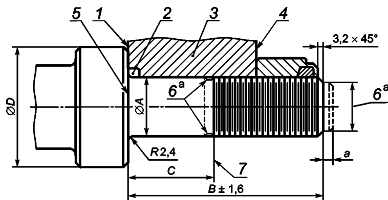
1 — заплечик N , заплечик плунжера, торец штока; 2 — необходимое уплотнение, размеры выбираются по усмотрению производителя; 3 — плунжер; 4 — заплечик P , заплечик плунжера, конец резьбы; 5 — заплечик M , заплечик штока; 6 — спад затылка на резьбе, конфигурация по усмотрению производителя; 7 — калибровочная часть резьбы; a — дополнительная возможность удлинения
