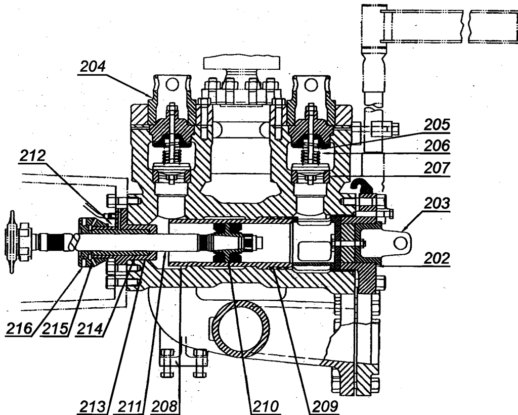
Рисунок В.4 — Нагнетательная часть дуплексного бурового насоса двукратного действия (номенклатуру деталей см. в таблице В.2)
