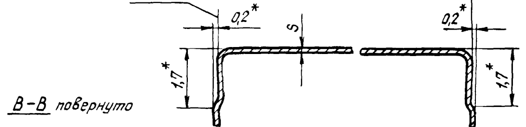
B-B
