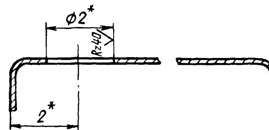
B-B повернуто
