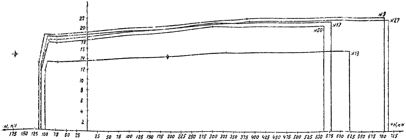
Диаграмма предельных нагрузок на фундамент п-3 из подмажников ФР-2 для различных грунтовых условий (ветровой режим)
