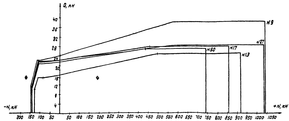
Диаграмма предельных нагрузок на фундамент П-Б из подожников ФЗ-2 для различных грунтовых условий (ветровой режим)
