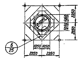
3-3 Горизонтальное опирание газоотводящего ствола
