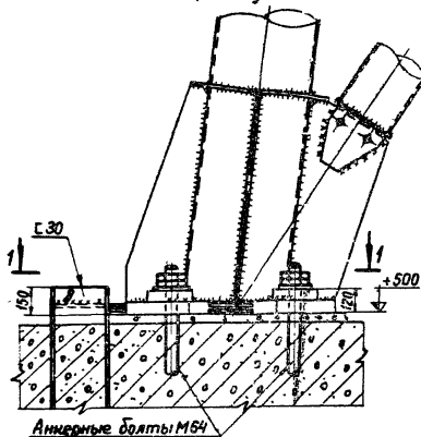
Опорный узел (2-2)
