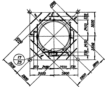
Вертикальное опирание газотводящего ствола на время ремонта
