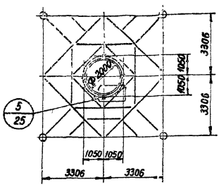
2-2 Вертикальное опирание газоотводящего ствола на время ремонта
