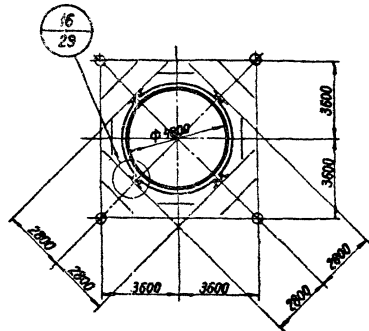
Горизонтальное опирание газотводящего ствола
