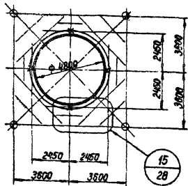
Вертикальное и горизонтальное опирание газотводящего ствола
