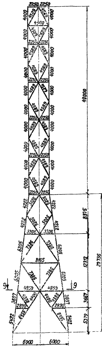
Геометрическая схема башни Развертка грани
