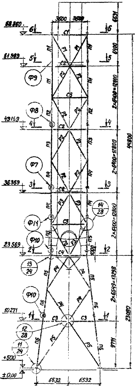
Схема сечений и усилий башни
