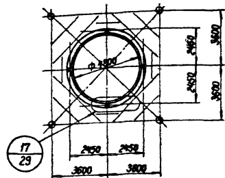
Вертикальное опирание газотводящего ствола на время ремонта
