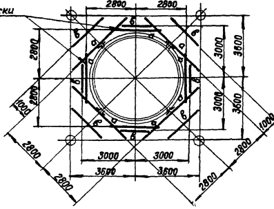
Горизонтальное опирание газотводящего ствола
