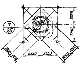
3-3 Горизонтальное опирание газоотводящего ствола
