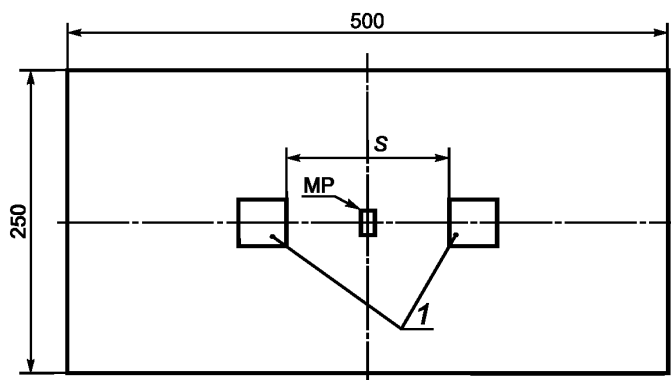
MP — точка измерения тангенциальной составляющей напряженности поля; s — расстояние между полюсами; 1 — полюса
