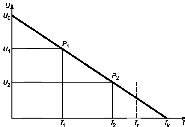
Рисунок 2 — Нагрузочные характеристики генераторов тока
