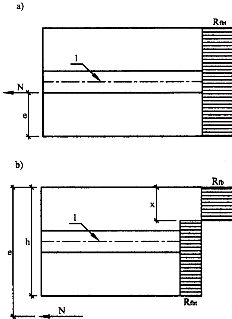
Рис.7. Эпюры напряжений во внецентренно растянутых элементах прямоугольного сечения а – при приложении продольной силы N в пределах ядра сечения; б – то же, за пределами 1 – стержневая или проволочная арматура
