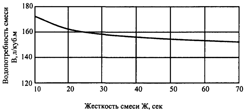
Рис. 3 График водопотребности пластичной (а) и жесткой (б) бетонной смеси
