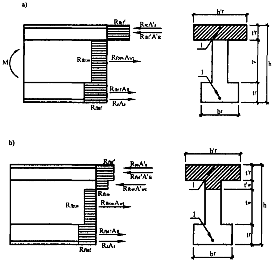
Рис.4. Схема распределения усилий и эпюра напряжений в сечениях, нормальных к продольной оси изгибаемого элемента двутаврового сечения при комбинированном армировании а – при \chi \leq \chi_r , б – при \chi > \chi_r
