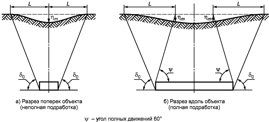
Рисунок С.1 — Основные параметры мульды сдвигения
