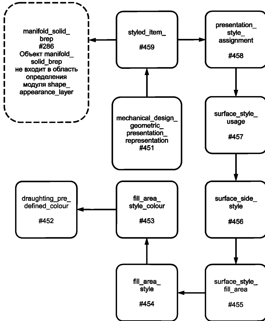
Рисунок F.4 — Задание цвета геометрической модели
