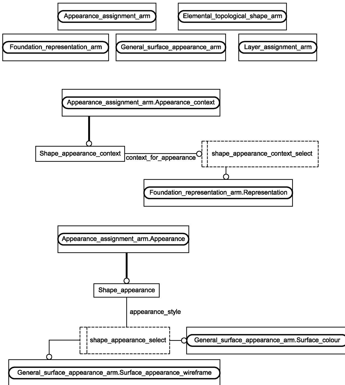
Рисунок С.1 — EXPRESS-G диаграмма ПЭМ
