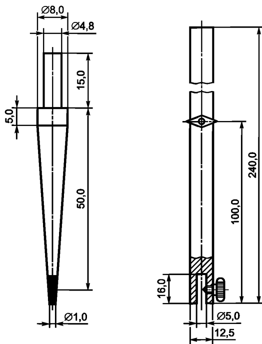
а) Съёмный конус, материал — сталь
