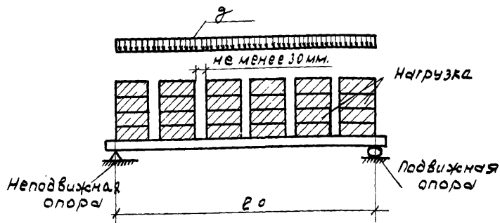
Схема нагрузки
