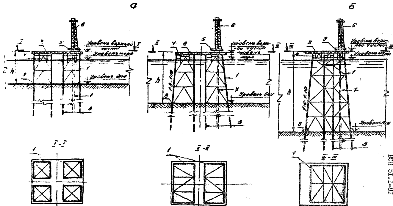
Рис. 1 Основные виды конструкций МНТС: а - многоблочные, б - одноблочные 1 - опорный блок, 2 - верхнее строение, 3 - свайный фундамент, 4 - причально-посадочное устройство, 5 - подрыльчатые конструкции, 6 - буровая вышка, 7 - обсадная колонна, 8 - опорный узел
