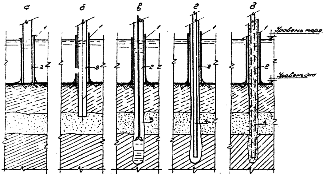
Рис. 5 схема устройства бурозаливной свай
