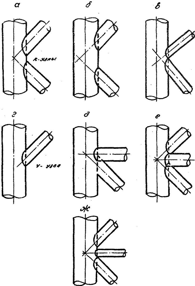
Рис. 3 Основные конструкции бесфланцевых узлов из труб
