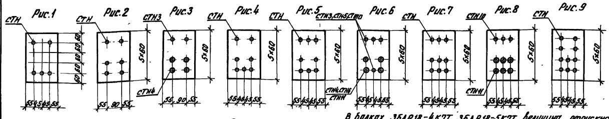
Расположение напрягаемой арматуры нижнего пояса в балках 1 типоразмера (16ДР18), поз.17
