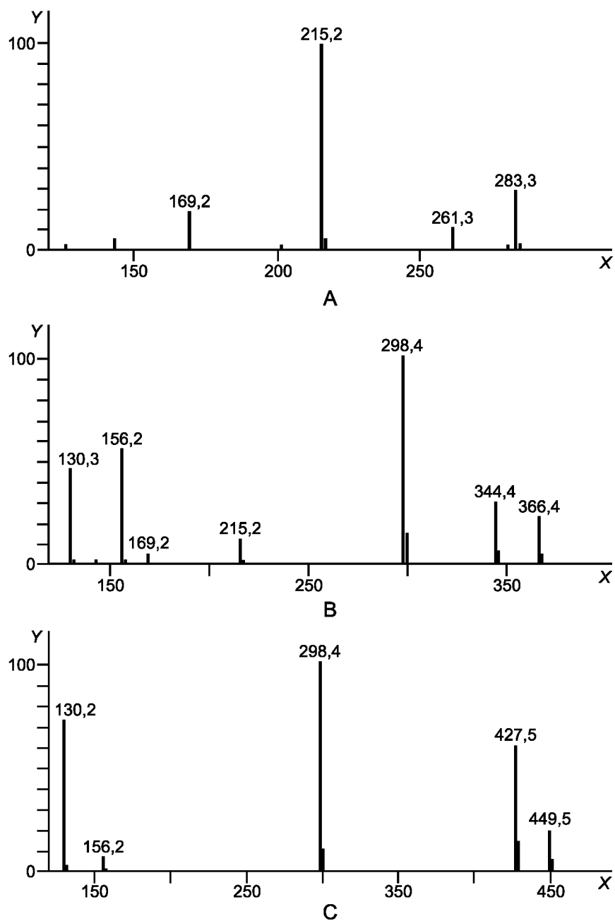
Рисунок В.4 — Масс-спектры с указанием относительной интенсивности для ЭТ-производного HAD (А), ЭТ-ДБА-производного HAI (В) и ДБА-производного HDI (С), полученные методом жидкостной хроматографии с использованием масс-спектрометрического детектора с электроспреем
