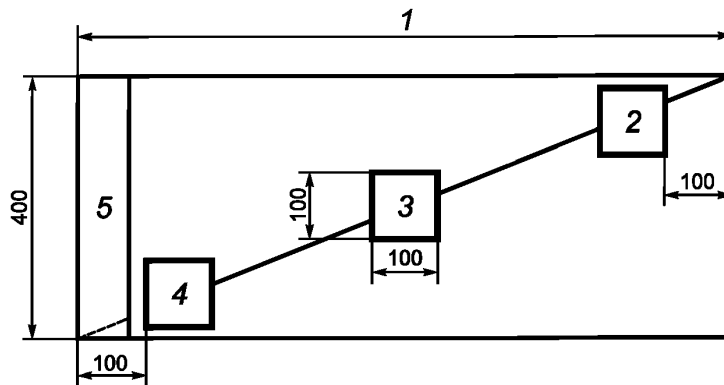
Рисунок 1 — Схема вырубki квадратных образцов
