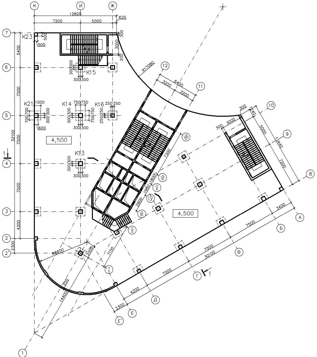
Рис. 1. План II этажа на отм. 4.500.
