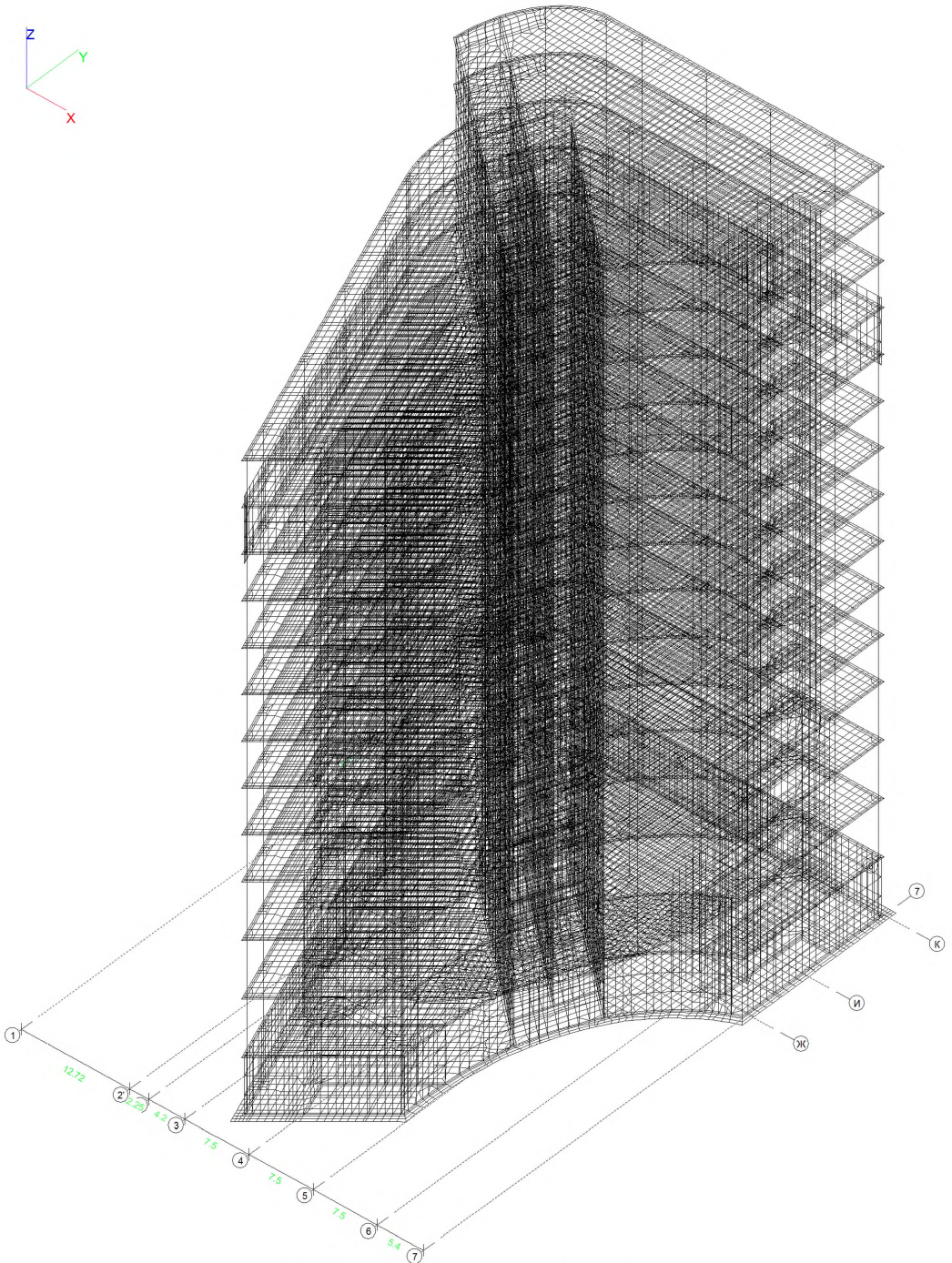
Рис.3. Расчетная схема каркаса здания.
