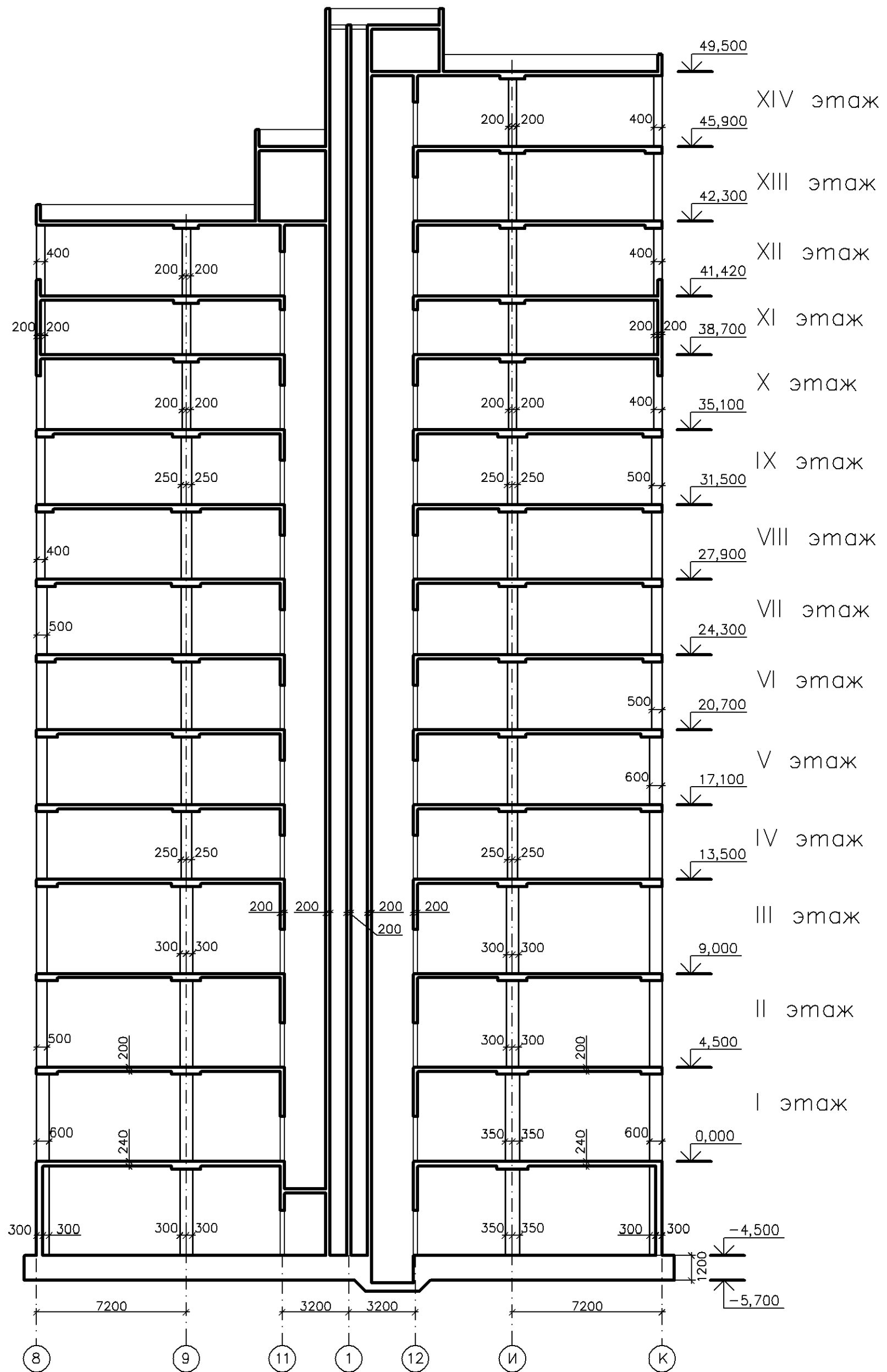
Рис.2. Разрез 1-1.
