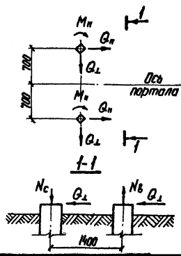
Схема нагрузок (шинный портал)
