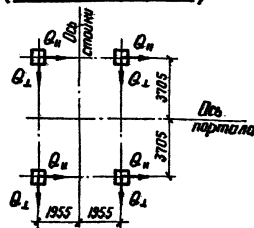
Схема нагрузок (ячейковый портал)
