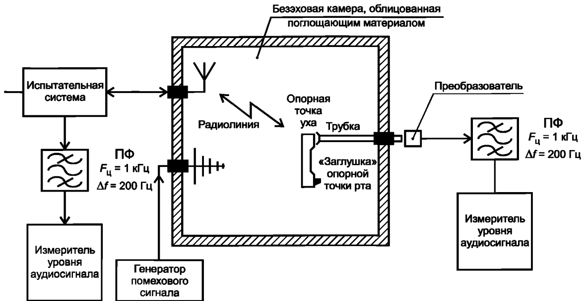
Рисунок 2 — Схема прохождения сигнала при испытаниях радиооборудования
