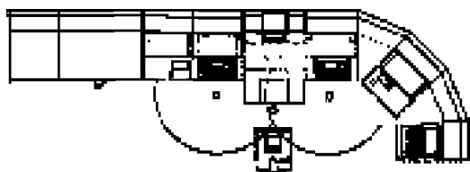
Рис. 2.7.3-2 Модифицированная конфигурация рабочего поста, базирующаяся на тех же принципах, которые показаны на рисунке 2.7.3-1.
