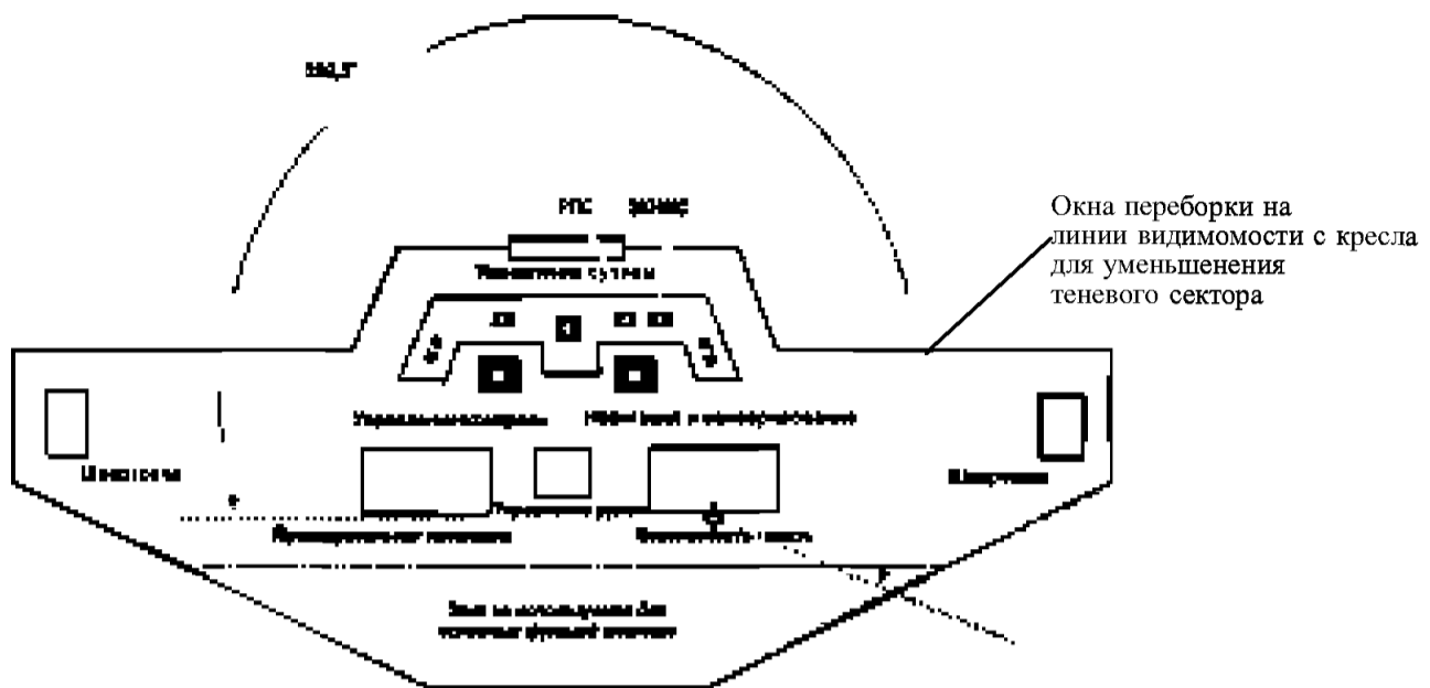
Рис. 2.5.17-2 Требуемая зона видимости с поста радиосвязи, во время контроля и эпизодического кратковременного использования оборудования ГМССБ вахтенным помощником Судовождение с использованием системы электронных карт (ЭКНИС) – место управления судном на пульте
