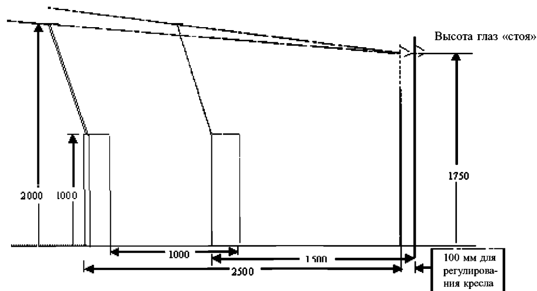
Рис. 2.6.3 При наклоне передних окон на угол 15^\circ от вертикали, угол обзора 5^\circ выше горизонтали от уровня глаз стоящего человека, находящихся на высоте 1750 мм может быть обеспечен на расстоянии 2600 мм от фронтальной стенки (лобовой переборки) с учетом наличия прохода шириной 1000 мм перед пультами рабочего поста
