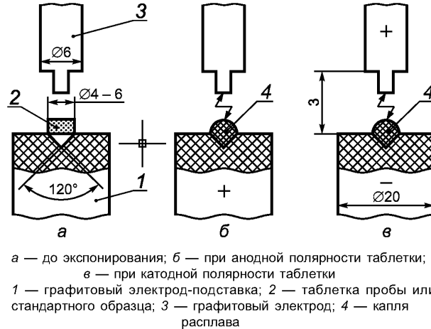
Рисунок 5 — Графитовые электроды
