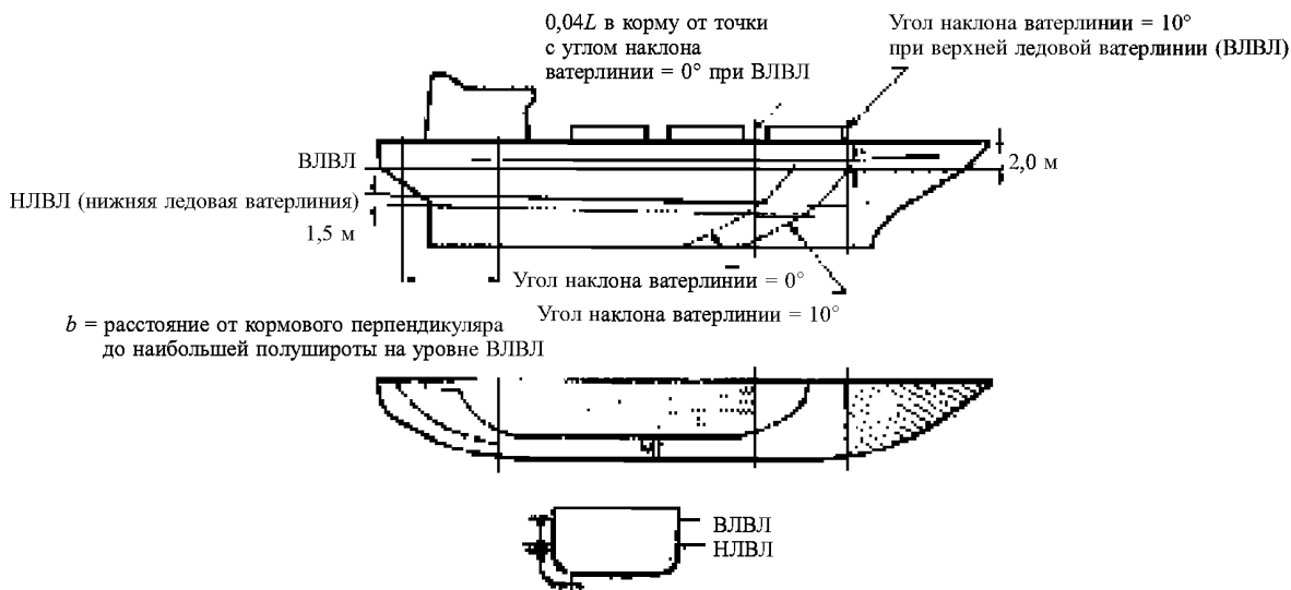
Рис. 1.2.2.1 Границы районов корпуса судна
