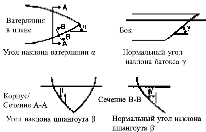
Рис. 1.2.3.2.1.1.1 Определение углов наклона
