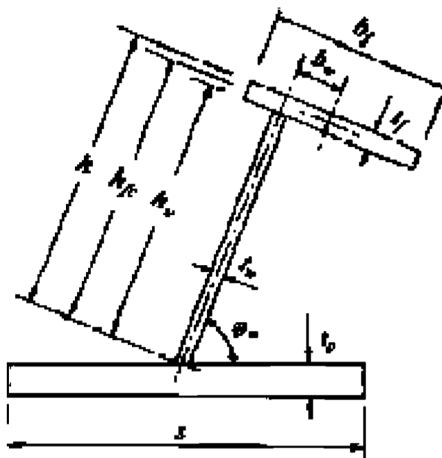
Рис. 1.2.5.7 Геометрия ребра жесткости
