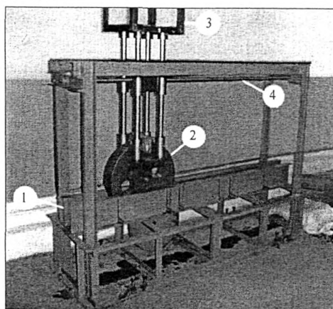
Рисунок Б VI.1 . Установка для уплотнения асфальтобетонной смеси:
