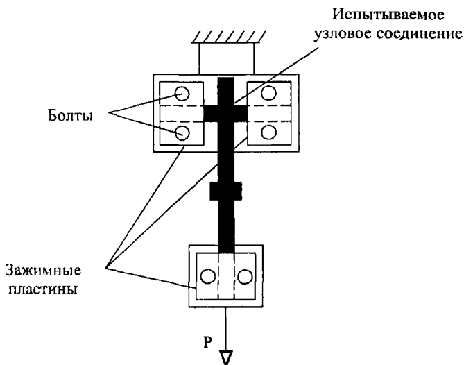
Рисунок Б 11 . Расчётная схема испытания на прочность узлового соединения ГМ
