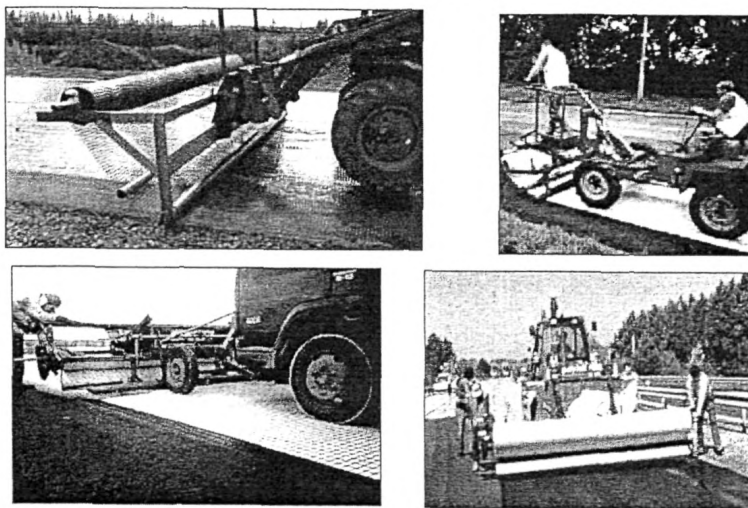
Рисунок 6. Навесные механизмы для раскладки армирующих материалов
