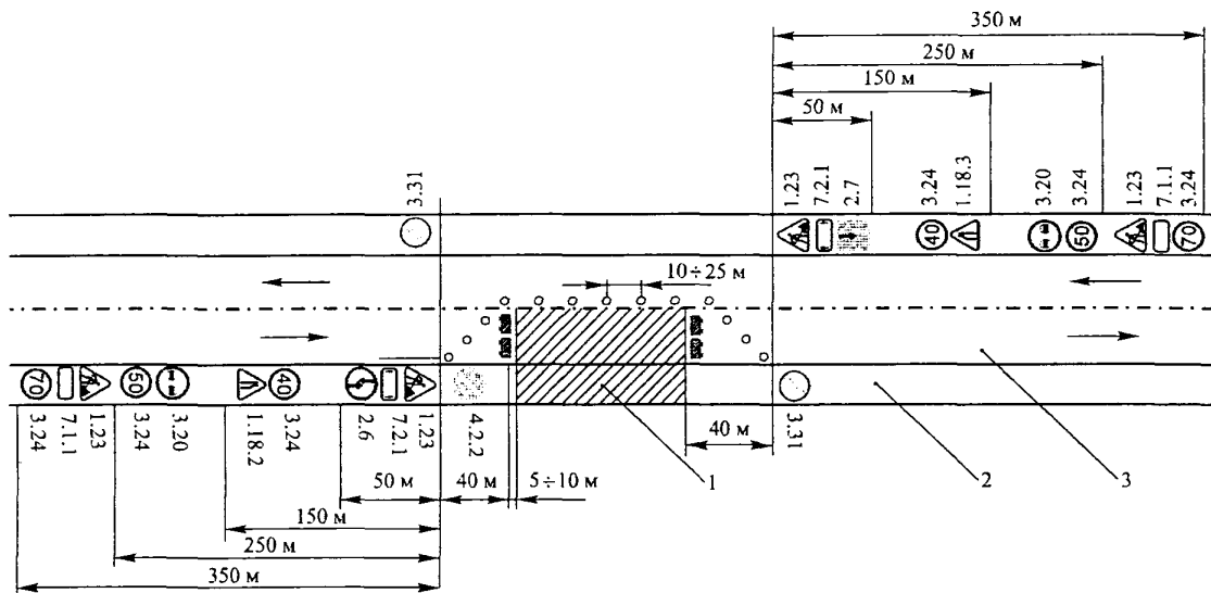
Рисунок 9. Организация ограждения места дорожных работ:
