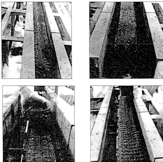
Рисунок Б VI.2 . Процесс извлечения геосетки из конструкции
