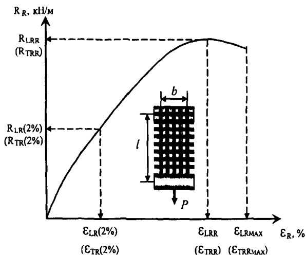
Рисунок Б 1.2 . График зависимости деформации от нагрузки
