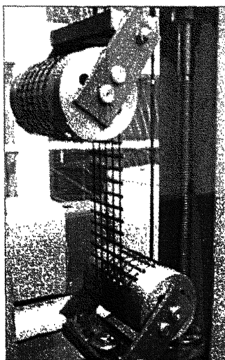
Рисунок Б 1.1 . Определение предела прочности ГМ при растяжении
