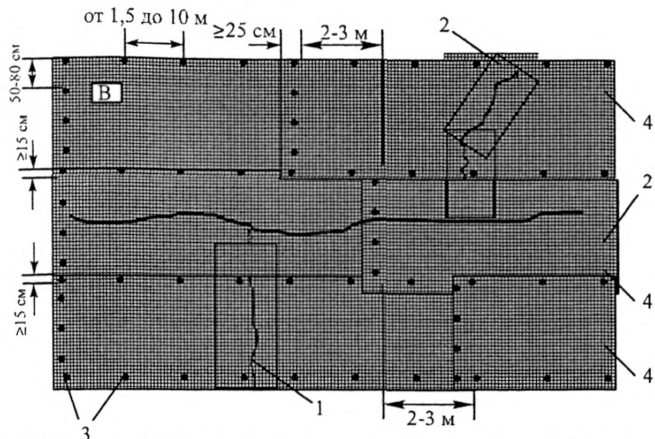
Рисунок 7. Схемы укладки и крепления полотен и полос геосетки на основании: А – при армировании сплошным полотном на кривых малого радиуса; Б – при армировании полосами над трещинами; В – при комбинированном армировании полосами и сплошным полотном; 1 – продольные и поперечные трещины; 2 – полосы геосетки; 3 – дополнительная фиксация полос к основанию; 4 – полотна геосетки, укладываемые поверх полос
