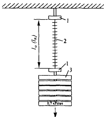
Рисунок Б V1 . Схема испытания ГМ на длительную прочность
