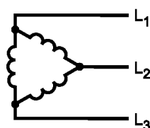
Соединение треугольником
