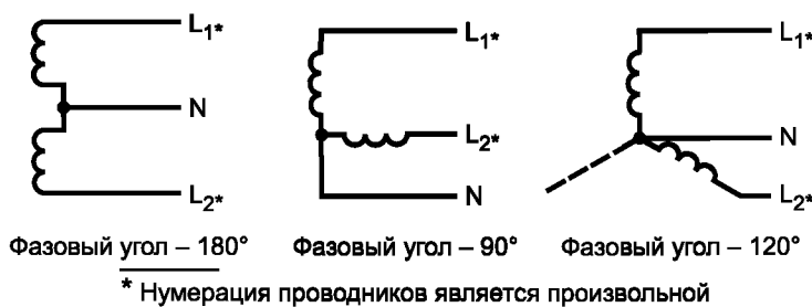
Рисунок 3 — Двухфазная трехпроводная система
