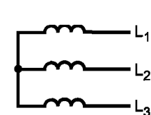
Соединение звездой
