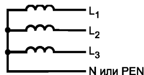
Рисунок 5 — Трехфазная четырехпроводная система
