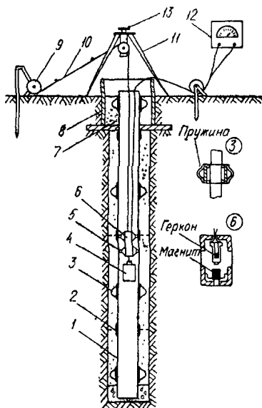
Рис. 45. Глубинная марка конструкции ВНИМИ
