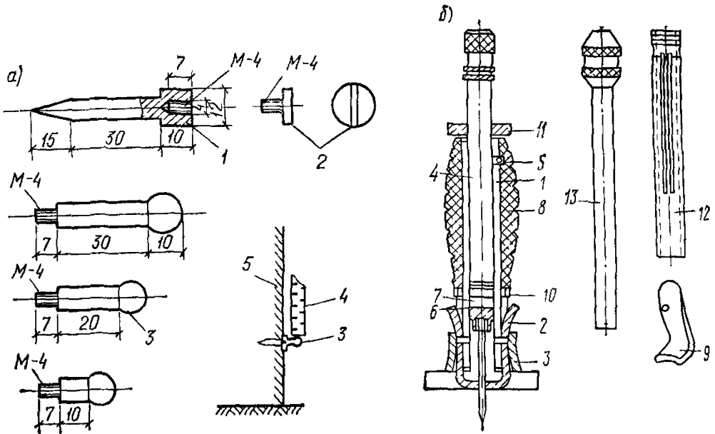
Рис. 39. Марка-дюбель
