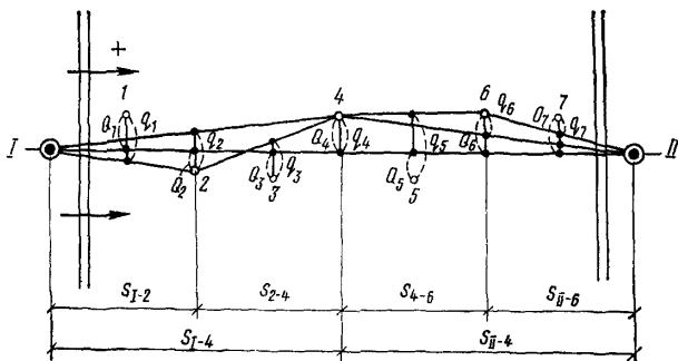
Рис. 10. Схема частей створа
