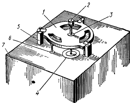
Тип Б (рис. 62)
