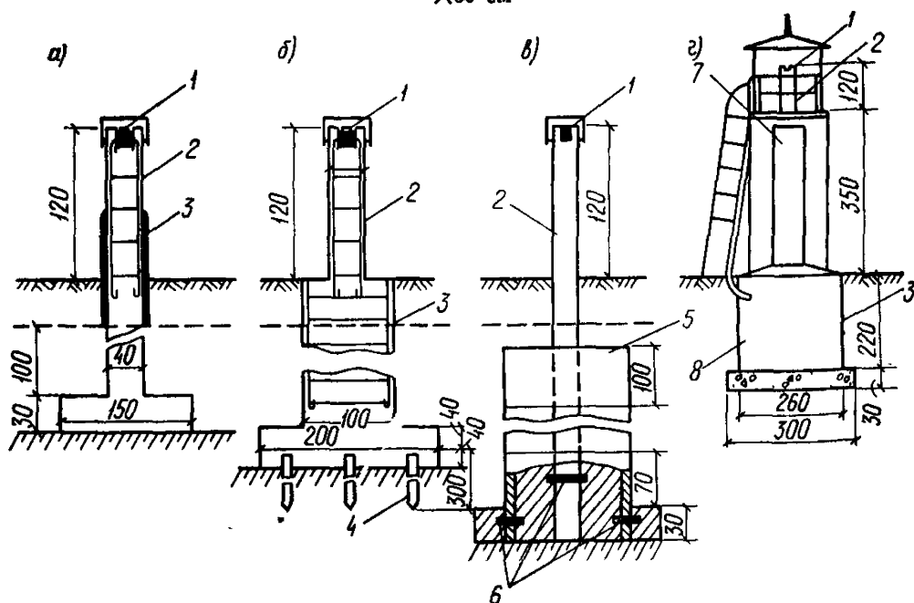
Рис. 60. Опорные знаки, выступающие над поверхностью земли
