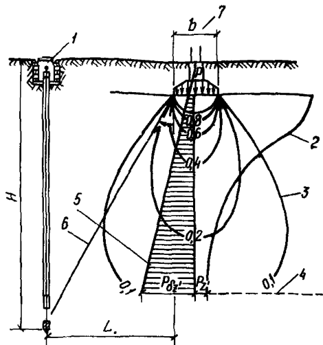
Рис. 2. Удаление грунтового репера от сооружения
