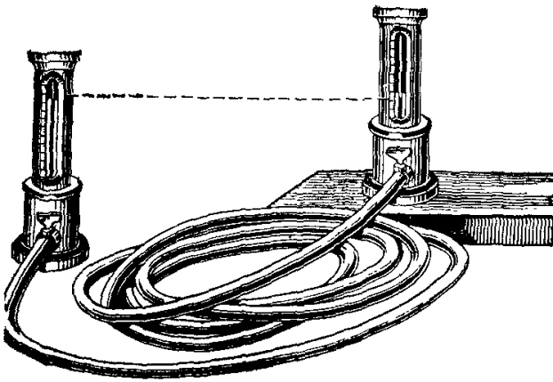
Рис. 52. Простейший гидростатический нивелир
