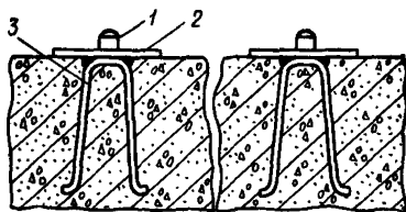
Рис. 73. Щелемер для длительных наблюдений 1 — марка; 2 — фланец; 3 — анкерная плита
