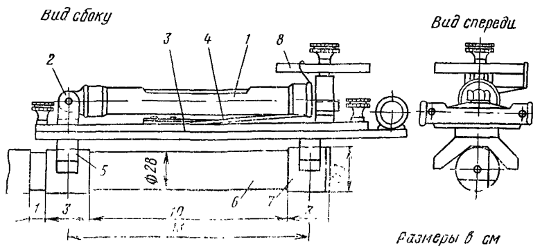
Рис. 23. Переносной клинометр 1 — уровень; 2 — шарнир; 3 — основание (устанавливается на измерительную базу); 4 — пружина; 5 — лагера; 6 — измерительная база; 7 — муфты
