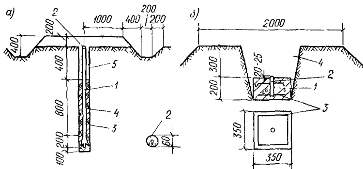
Рис. 28. Оползневые марки
