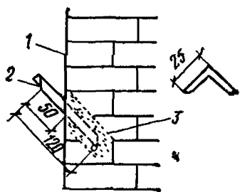
Рис. 31. Стенная марка (уголок)
