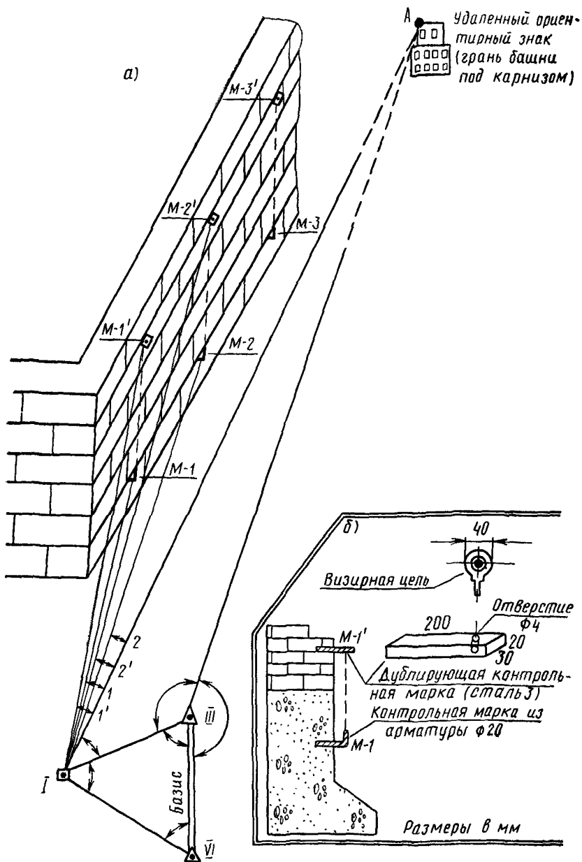
Рис. 18. Комбинированный метод для жилых зданий а — схема определения сдвига; б — конструкция и установка марок на здании I—VI — опорные знаки; M-1, M-2, M-3 — марки
