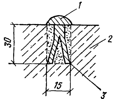
Рис. 37. Цокольная марка
