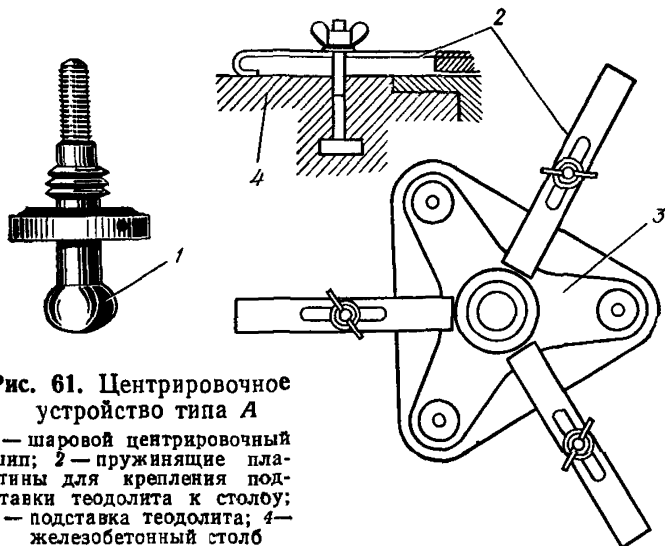
Тип А (рис. 61)
