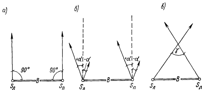
Рис. 16. Основные случаи съемки
