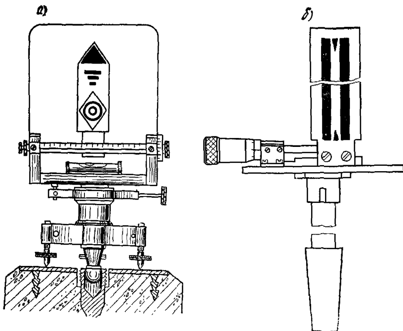
Рис. 65. Подвижные визирные цели
