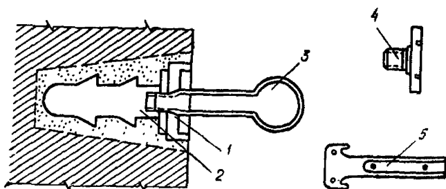
Рис. 32. Стенная марка закрытого типа
