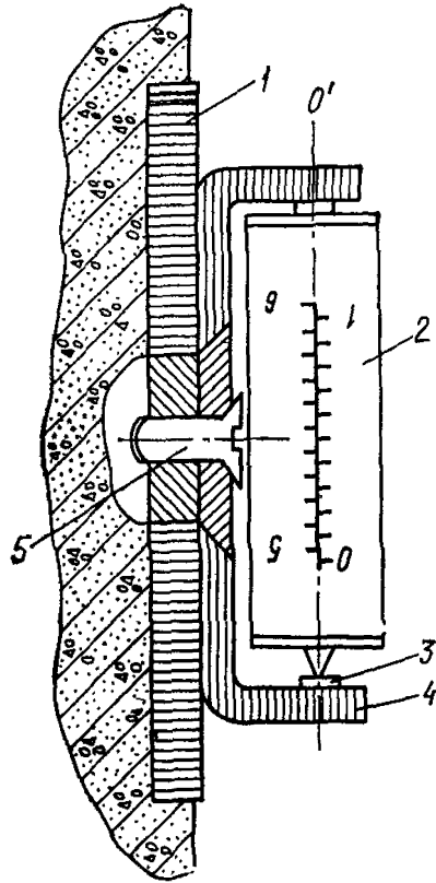
Рис. 35. Стенная марка конструкции М. Е. Пискунова
