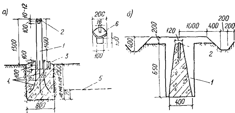
Рис. 27. Опорные знаки для наблюдений за оползнями
