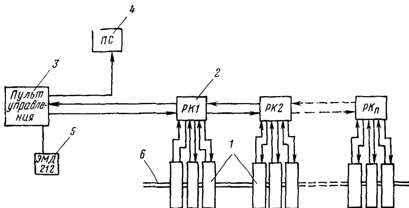
Рис. 58. Стационарная гидростатическая система с дистанционным съемом информации
