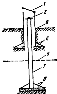
Рис. 42. Поверхностная грунтовая марка
