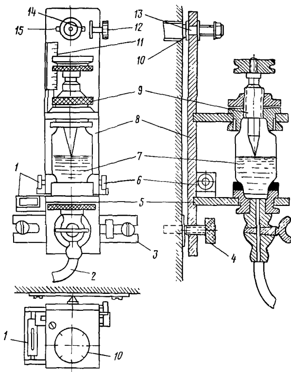
Рис. 54. Гидростатический нивелир института Унипроедь
