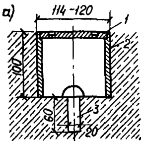
Рис. 36. Плитная марка
