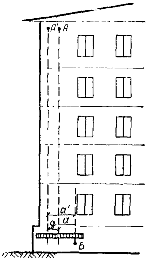
Рис. 21. Метод проектирования при измерении крена сооружения
