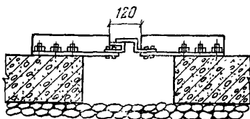
Рис. 74. Щелемер для измерения широких трещин и швов
