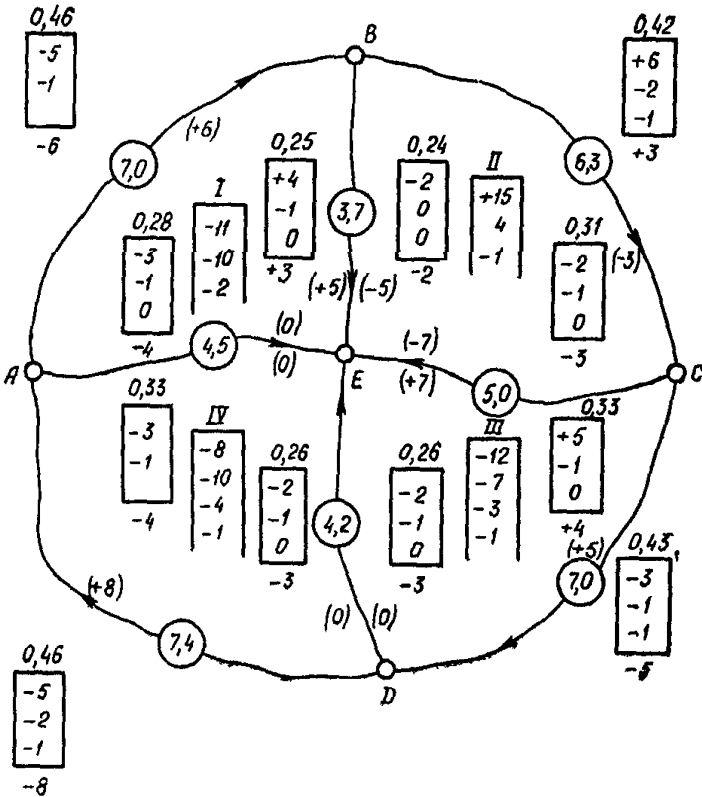
Рис. 50. Уравнивание способом полигонов
