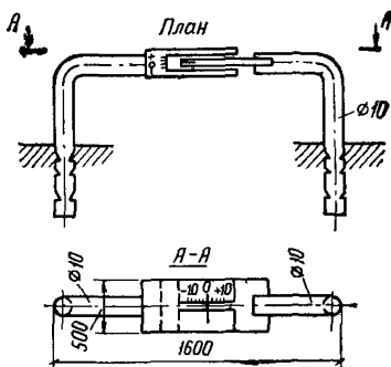
Рис. 69. Маяк из плексигласа
