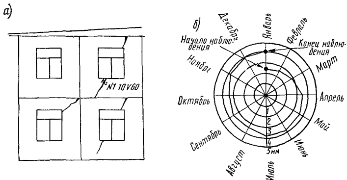
Рис. 26. Фиксирование развития трещин
