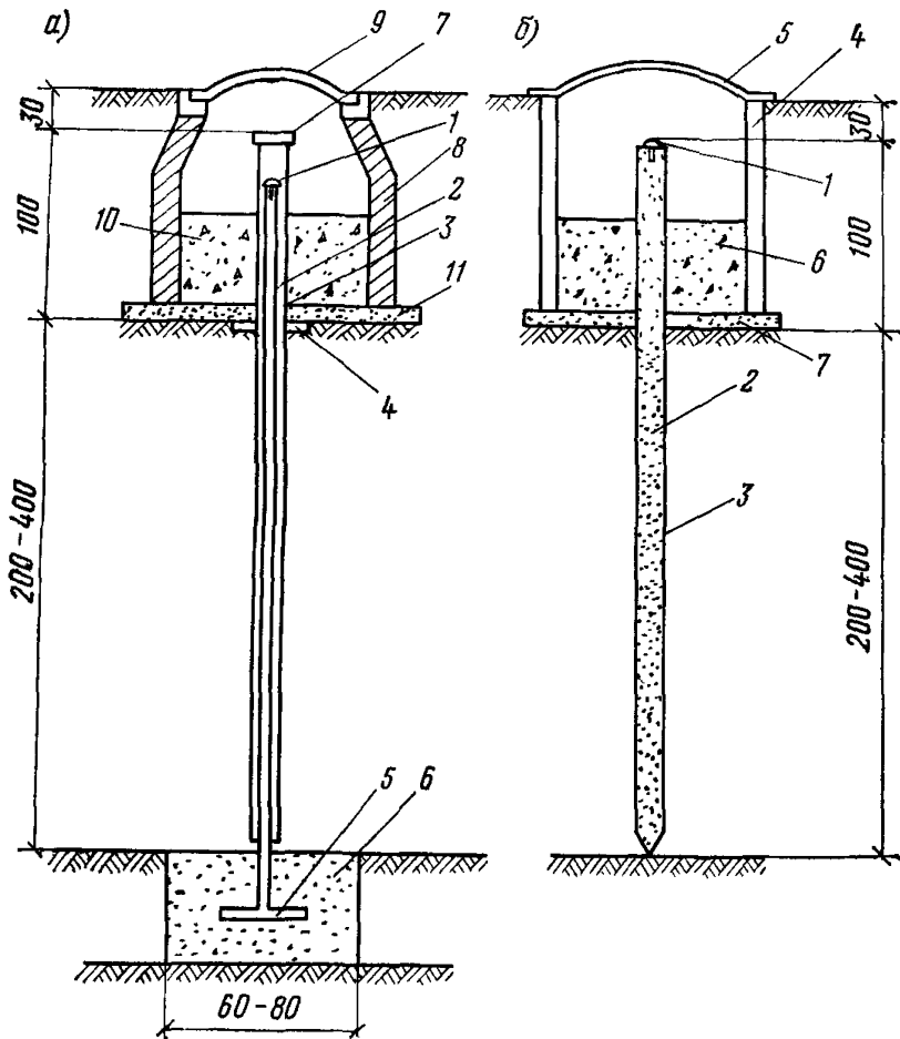
Рис. 3. Грунтовые реперы
