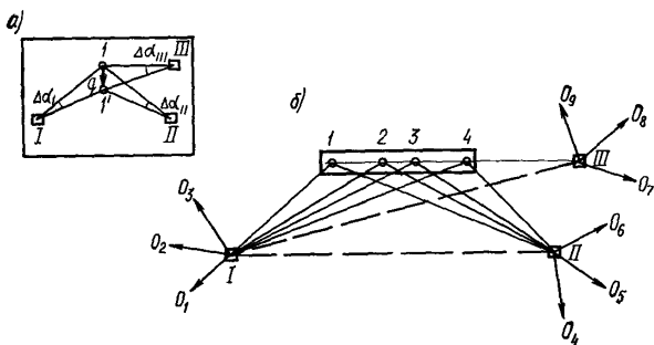
Рис. 13. Метод направлений
