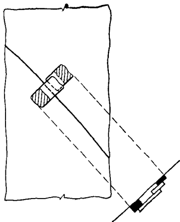
Рис. 70. Щелемер конструкции ЛенГИДЭПа
