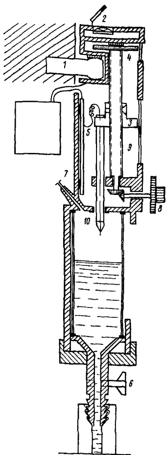
Рис. 57. Гидростатический нивелир Мейссера
