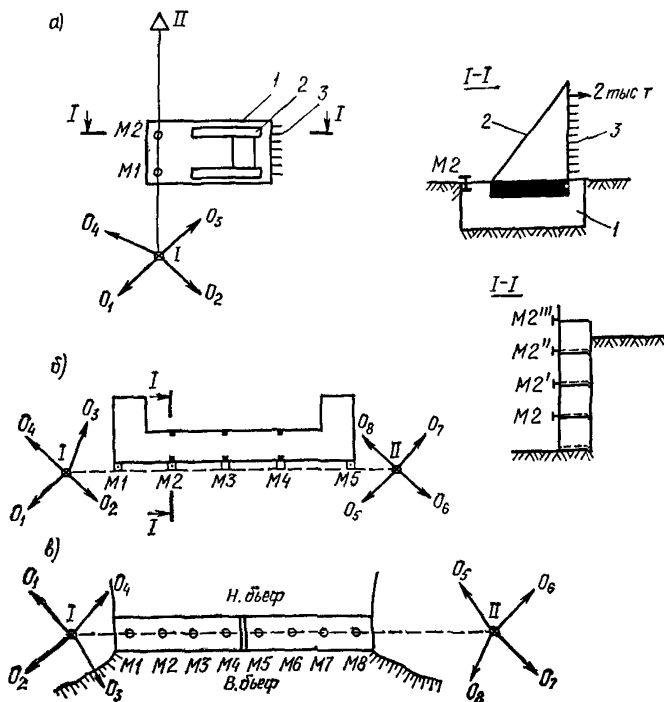
Рис. 9. Метод створа для разного рода сооружений
