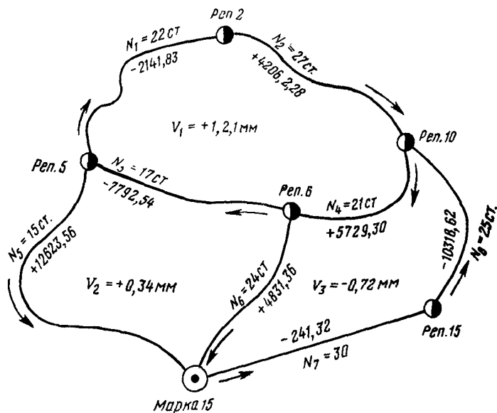
Рис. 51. Уравнивание способом наименьших квадратов
