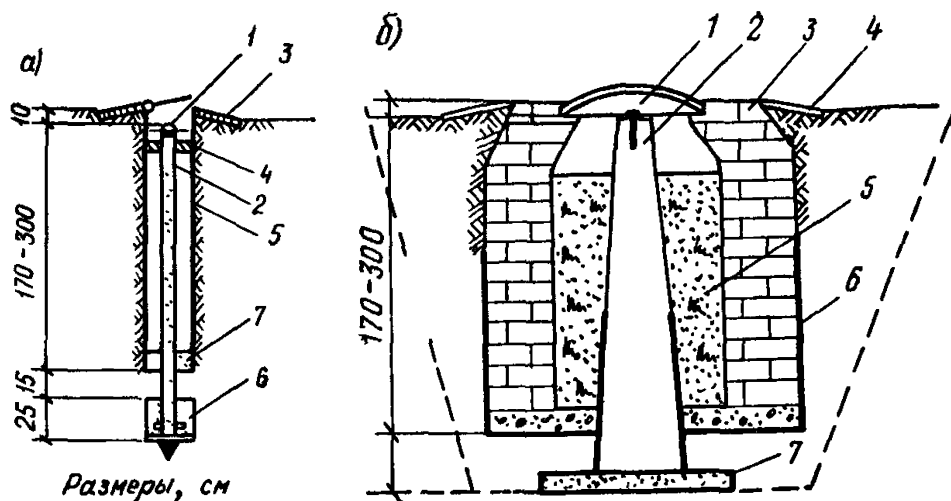
Рис. 59. Скрытые опорные знаки
