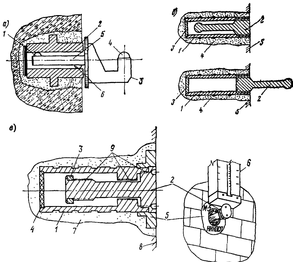
Рис. 33. Марки закрытого типа
