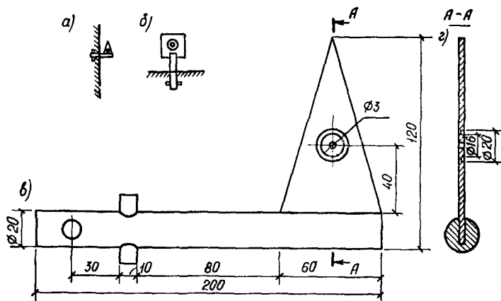
Рис. 67. Марки с визирными целями, наглухо устанавливаемые на сооружениях, рекомендуемые для метода направлений а и б—общий вид марок; в—вид спереди; г—разрез по А—А
