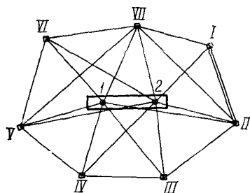
Рис 14. Метод триангуляции
