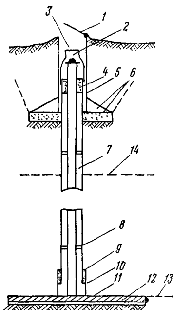
Рис. 41. Глубинная железобетонная плита-марка 1 — крышка; 2 — полусферическая головка; 3 — защитная крышка; 4 — сальник; 5 — защитная труба \varnothing 100—168 мм; 6 — металлический лист; 7 — рабочая труба \varnothing 50—100 мм; 8 — распорная диафрагма; 9 — сальник; 10 — выдвигаемое звено защитной трубы; 11 — металлический лист 1,5 \times 1,5 м; 12 — железобетонная плита 1,5 \times 1,5 м; 13 — основание; 14 — линия промерзания грунта
