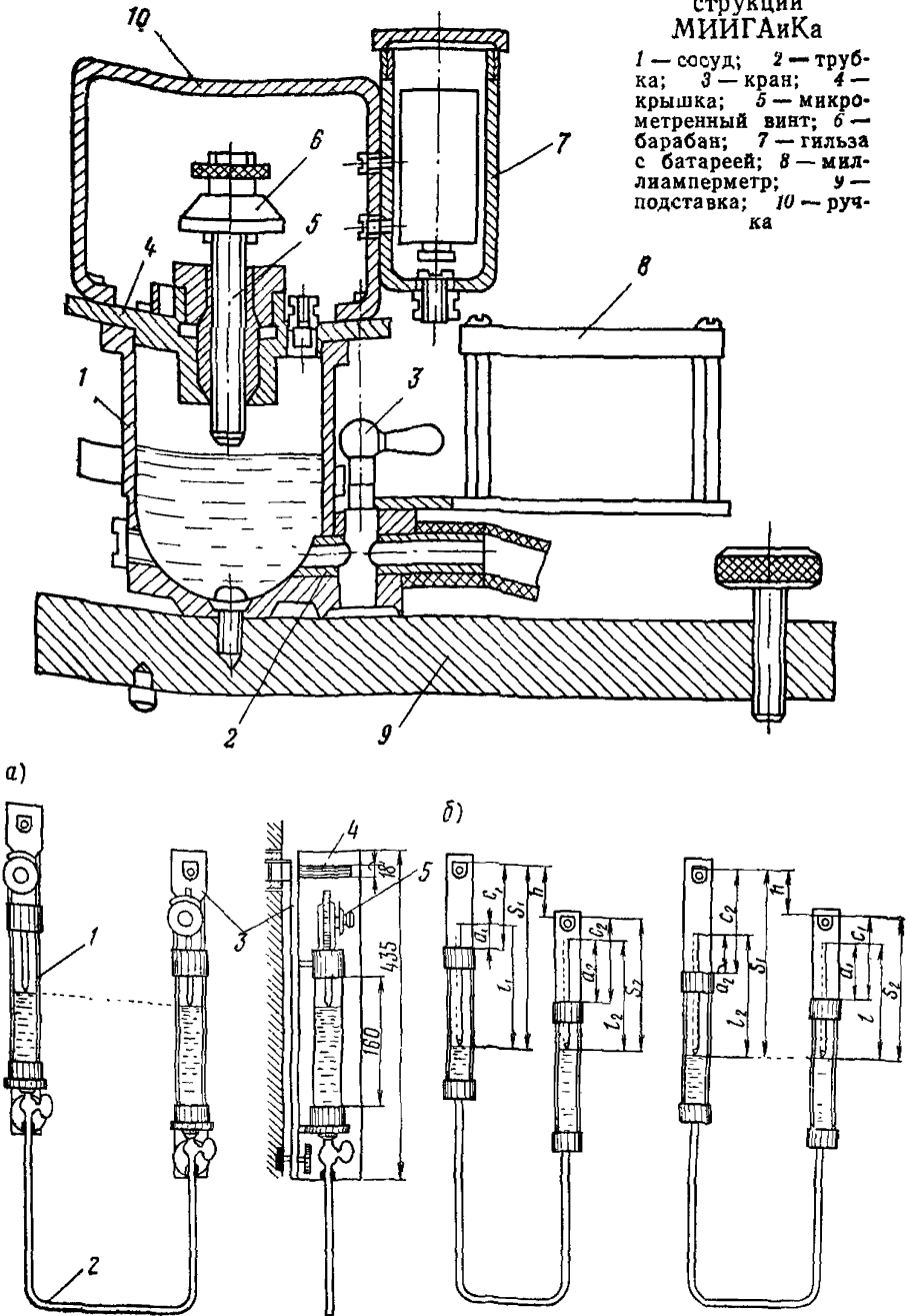
Рис. 56. Гидростатический нивелир Терцаги
