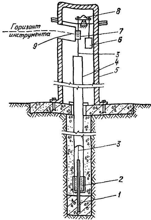
Рис. 1. Глубинный репер с гибкой реперной штангой
