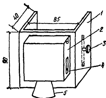
Рис. 48. Осветительная рамка 1 — корпус рамки 90×85×40 мм изготавливается из металла; 2 — футляр для электробатарейки, прикрепляется винтами к корпусу; 3 — винт для крепления рамки к рейке; 4 — выключатель; 5 — рефлектор с электролампочкой
