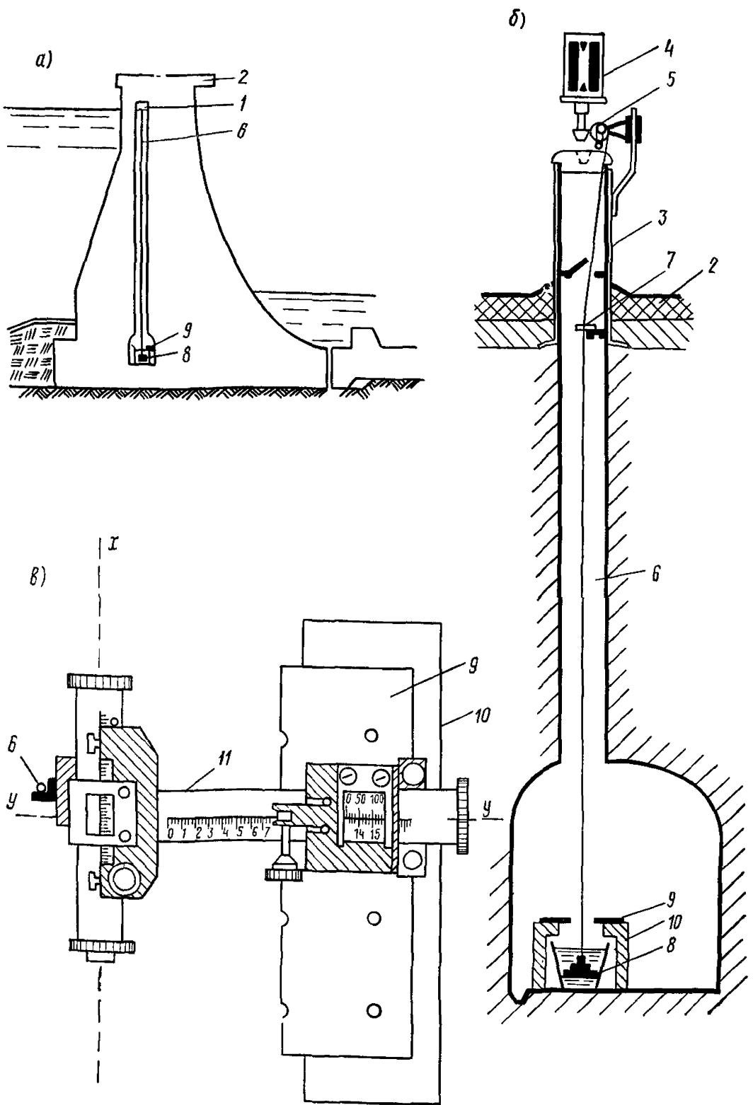
Рис. 24. Отвес конструкции Гидропроекта
