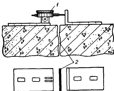
Рис. 72. Щелемер с мессурой 1 — мессура; 2 — трещина
