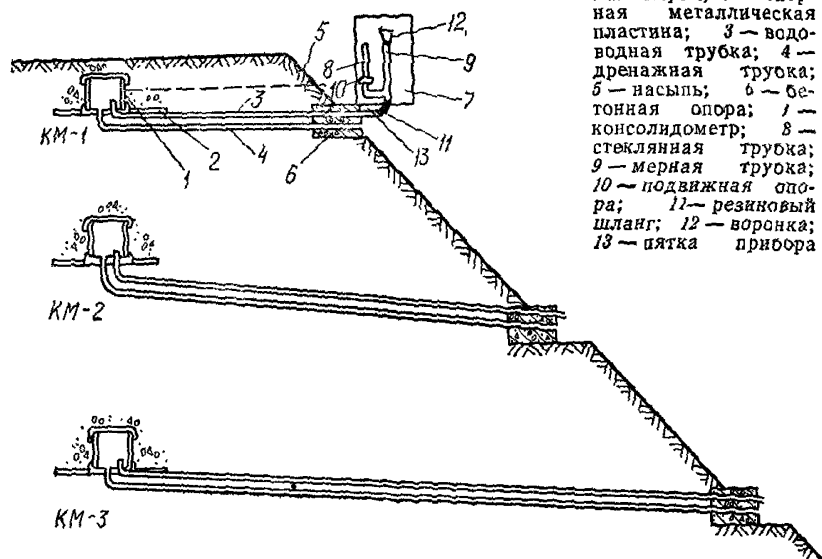
Рис. 43. Консолидометр
