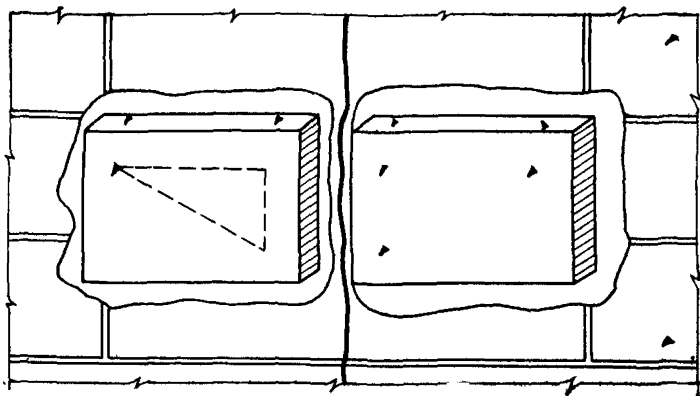
Рис. 71. Маяк конструкции Белякова
