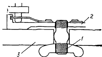
Рис. 64. Центрировочное устройство типа Г 1 — винт; 2 — подставка; 3 — знак
