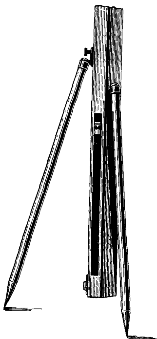
Рис. 6. Инварная штриховая рейка а — изображение рейки в поле зрения трубы нивелира Ni-002; б — рейка с подпорками для установки
