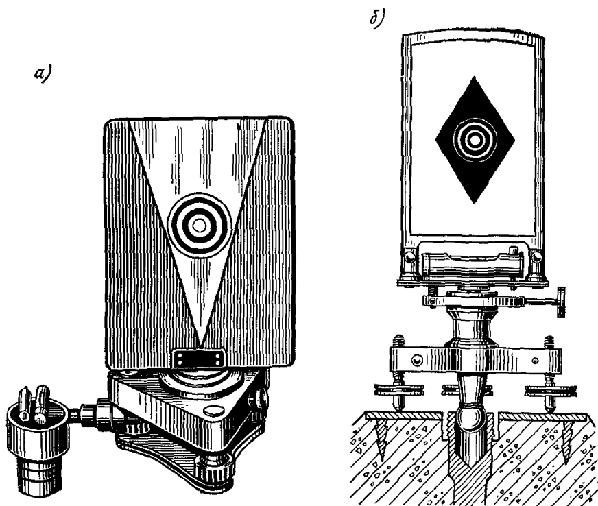
Рис. 66. Неподвижные визирные цели
