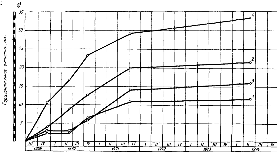
Рис. 20. График сдвига марок во времени а — график давлений; б — график сдвига
