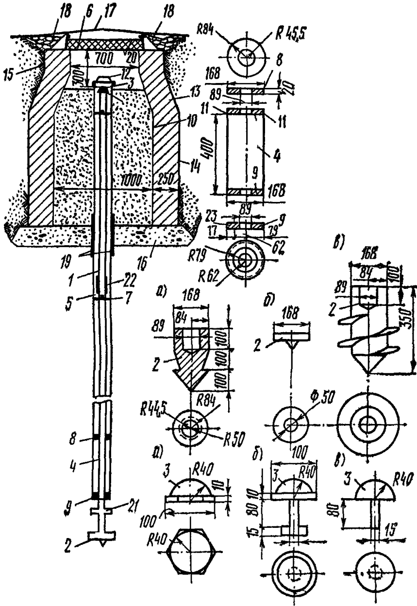
Рис. 30. Глубинный репер (общий вид и детали)
