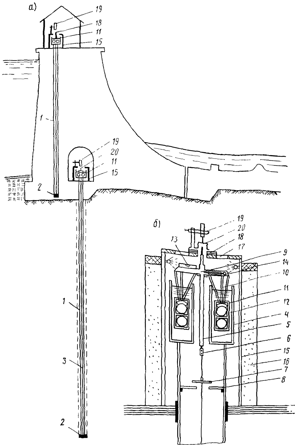
Рис. 25. Обратный поплавковый отвес
