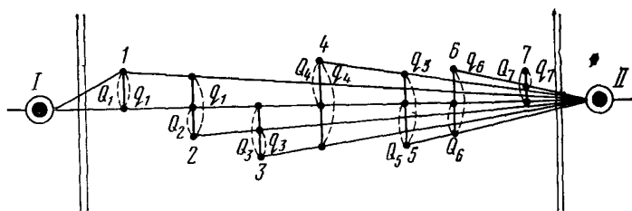
Рис. 11. Схема последовательных створов
