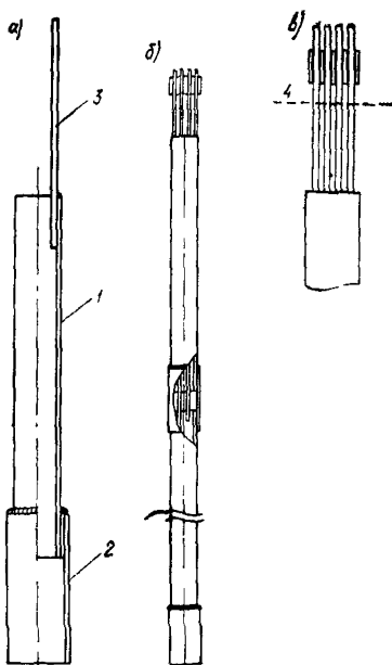
Рис. 46. Многоточечная глубинная марка
