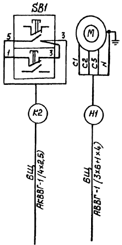
Схема подключения
