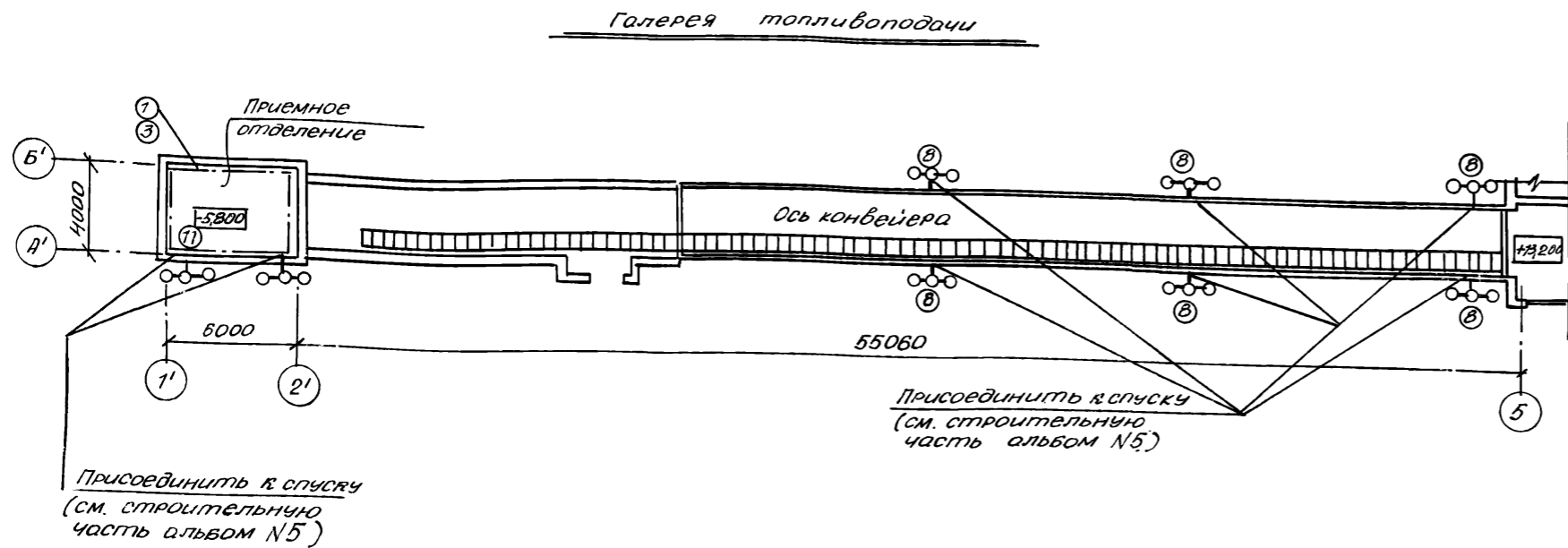
Надбункерная галерея
