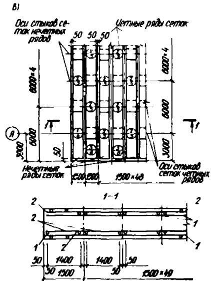
Рис. 69. Схема раскладки унифицированных сеток армирования прямоугольной плиты
