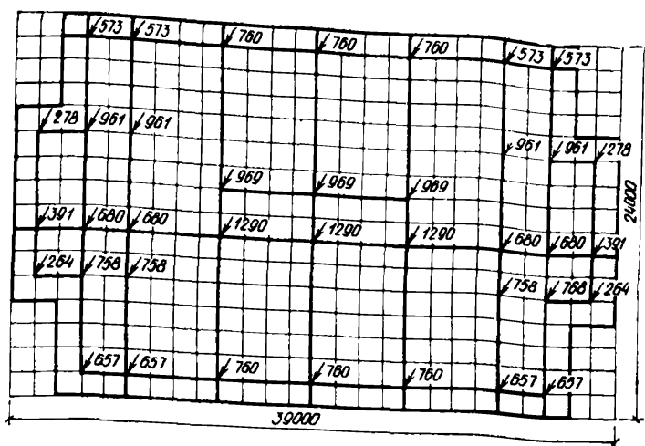
21. Схема плитного фундамента, рассчитанного на однородном и неоднородном основании
