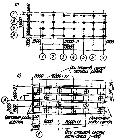
Рис. 69. Схема раскладки унифицированных сеток армирования прямоугольной плиты
