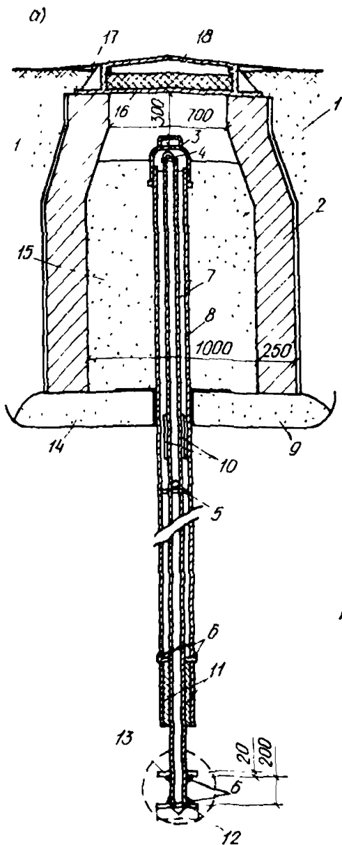
Рис. 75 Глубинный репер а — глубинный репер в сборе, б — стальная крышка защитной трубы, в — реперная головка, г — сальник
