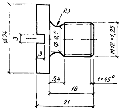
Рис. 72. Крышка стенной марки
