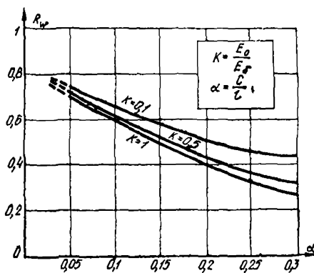
Рис. 39. Коэффициент перехода R_w
