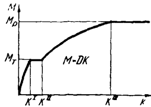
Рис. 66. Диаграмма деформирования железобетона
