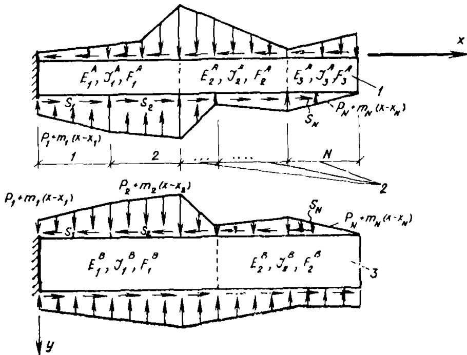
Рис. 53. Схема здания контактных напряжений на горизонтальных разрезах 1 — слой А, 2 — участки контакта, 3 — слой В
