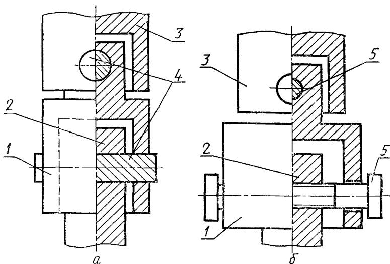
Рис. 5. Шарнир Гука:
