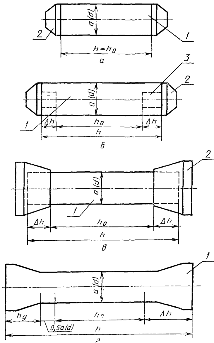
Рис. 1. Расположение зон однородного напряженного состояния ( h_0 ) и влияния захватов \Delta h при испытаниях с использованием приклеиваемых (а), анкерных (б), цапговых (в) захватов и на образцах с галтелями (г)
