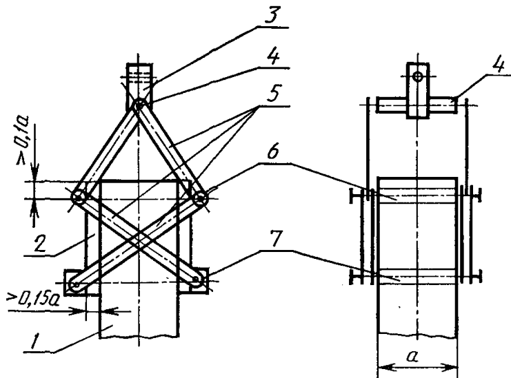
Рис. 4. Схемы съемного самозажимного захвата для образцов-призм:
