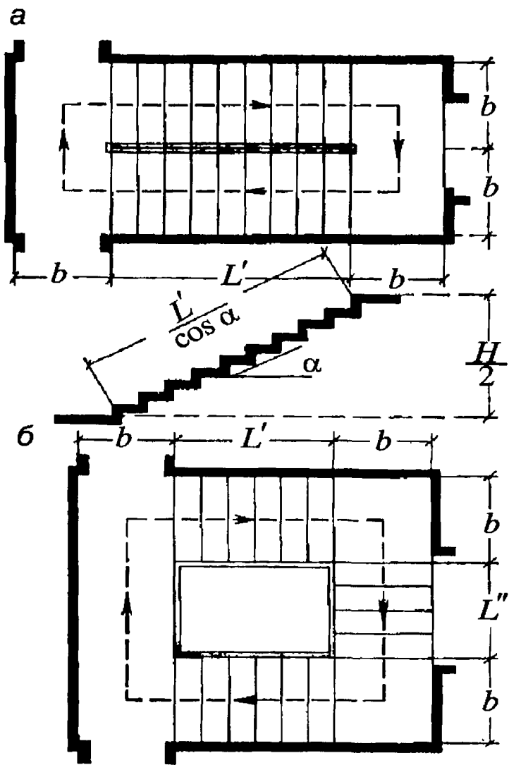
Рис. П5.1. Расчетная длина пути по лестнице: а – двухмаршевая лестница; б – трехмаршевая лестница
