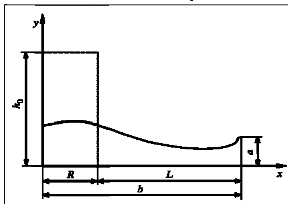
Рис. П3.2. Типичная картина движения жидкости в обваловании при квазимгновенном разрушении резервуара: --- - уровень начального столба жидкости; ——— - уровень жидкости в промежуточный момент времени (результаты расчета)
