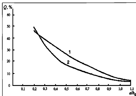
Рис. П3.3. Зависимость доли перелившейся через обвалование жидкости Q от параметра ah_0 : 1 - расчет; 2 - эксперимент
