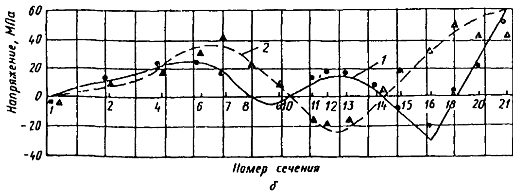
а — меридианные напряжения; б — окружные напряжения; 1, 2 — по теории оболочек на внутренней и наружной поверхностях соответственно; ●, ▲ — решение осесимметричной задачи теории упругости для внутренней и наружной поверхностей
