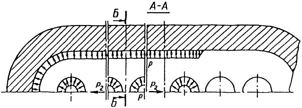
Расчетная схема корпуса блока регулирующих клапанов
