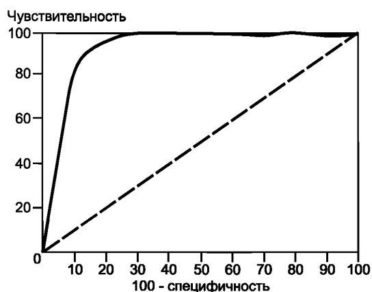
Рисунок 3 — ROC-кривая
