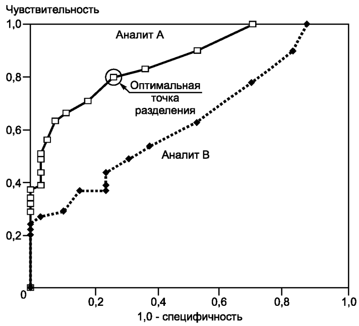
Рисунок 4 — Сравнительная оценка ROC-кривых двух аналитов
