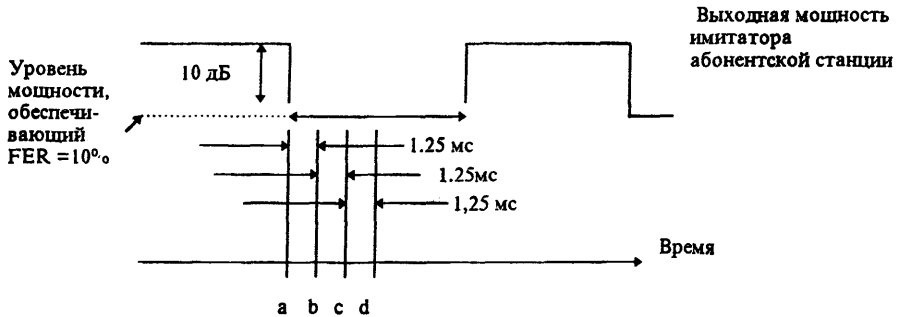
Рис.5.2.4-1 Интервалы команд увеличения мощности АС
