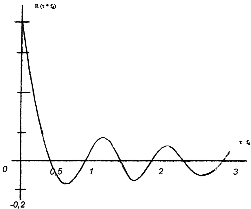
Рис.1.2.1. Функция автокорреляции фазы
