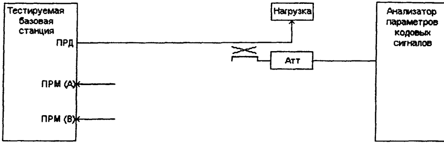
Рис 1.1 10 Схема измерения параметров кодовых сигналов
