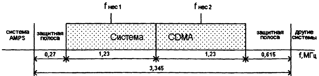
Рис. 2.2. Полоса частот, занимаемая системой CDMA, для случая двух несущих.
