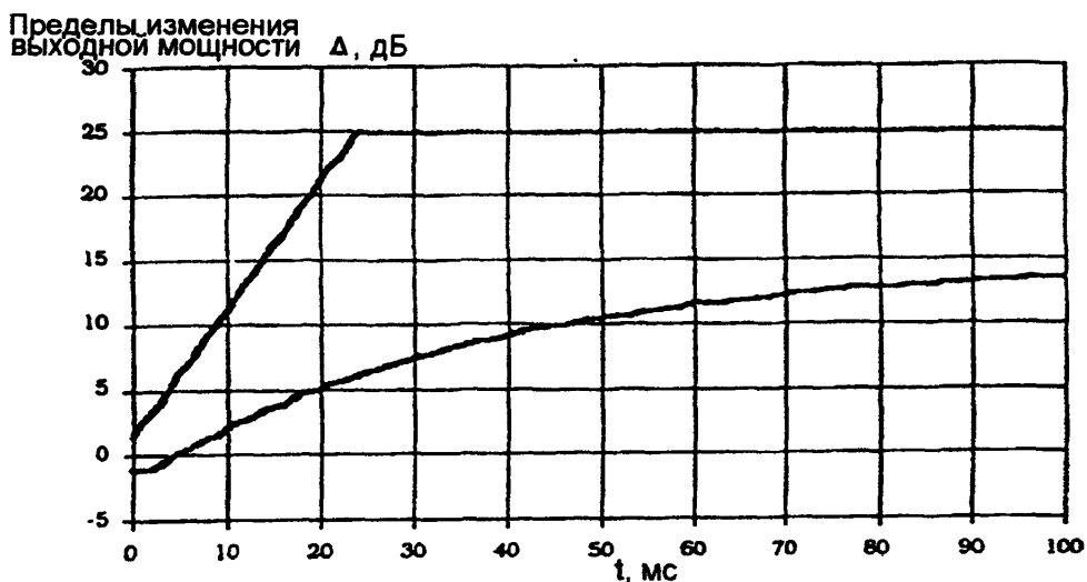
Рис.4.2.4.2.1. Шаблон изменения выходной мощности при \Delta P_{\text{в}}=20 дБ
