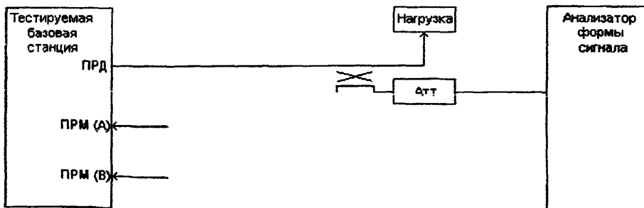
Рис 1.1.9. Схема измерения качества формы сигнала
