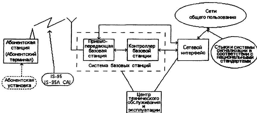
Рис.3. Конфигурация системы радиотелефонной связи стандарта CDMA
