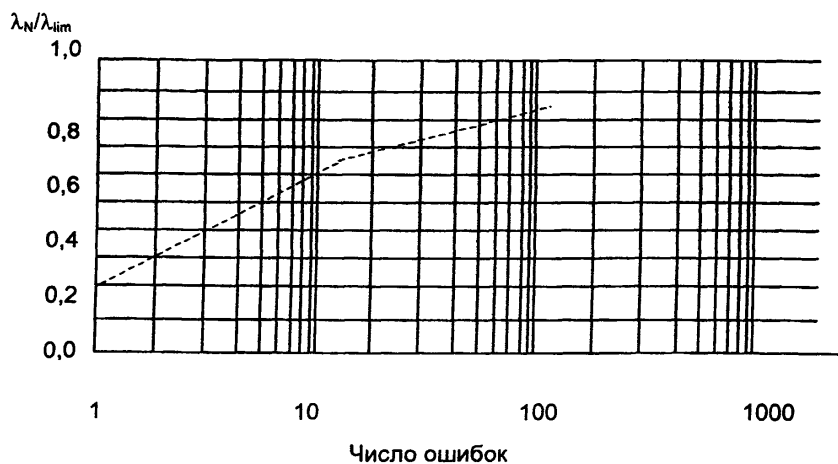
Рис.1 Зависимость допустимого значения \lambda_N/\lambda_{lim} от числа ошибок К для доверительной вероятности 95%
