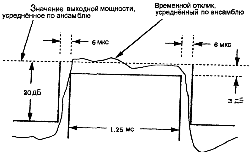
Рис.4.2.4.7. Шаблон огибающей мощности передатчика.
