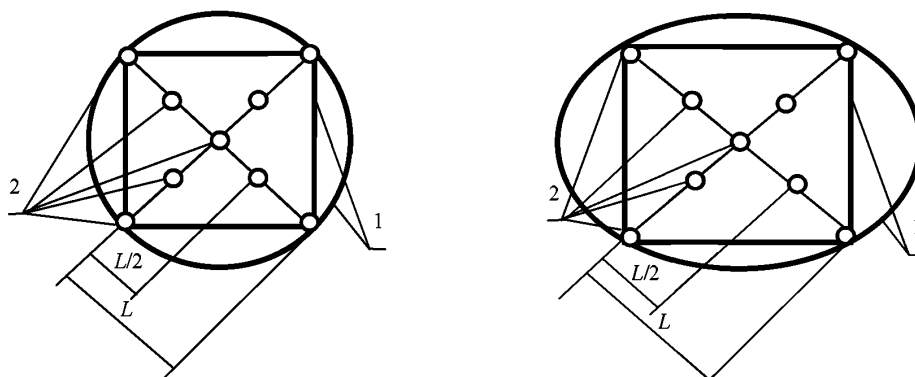
L — радиус (половина диагонали) защищаемой площади; 1 — граница защищаемой площади; 2 — модельные очаги
