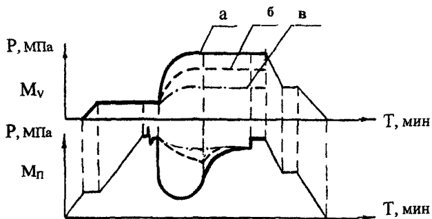
Рисунок 1.2.7 Диаграммы изменения давления на забое ( M_{п} ) и в трубах ( M_v ) при испытании высокопродуктивных пластов с различными диаметрами штуцеров ( d_{ш}^a > d_{ш}^б > d_{ш}^в )
