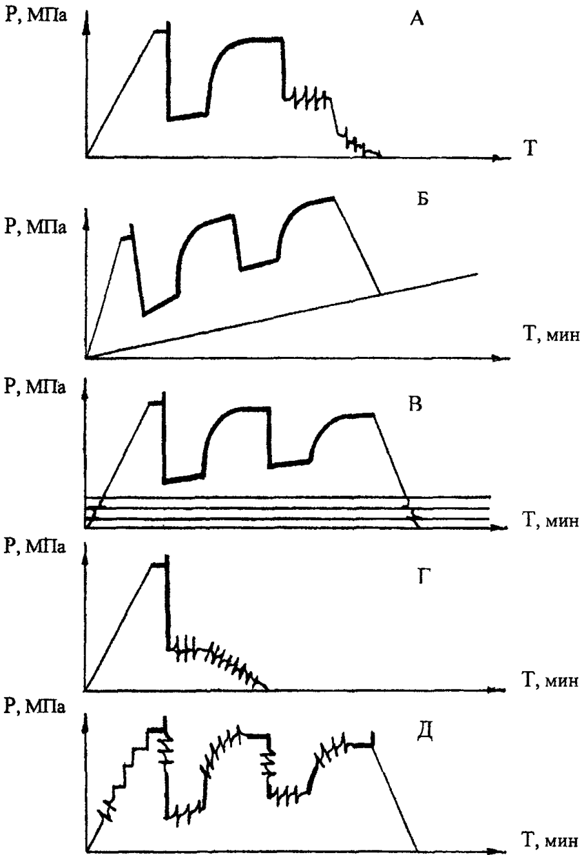
Рисунок 1.2.1 Примеры диаграмм, зафиксированные при плохой технической подготовке скважинных манометров.
