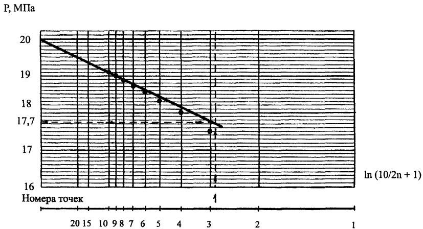
Рисунок 2.1.2 Палетка обработки КВД с шагом расшифровки \Delta t = 0,2T
