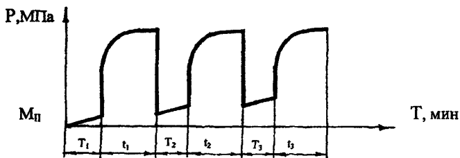
Рисунок 1.1.4 Диаграмма изменения давления манометра M_{II} многоциклового испытания пласта средней активности
