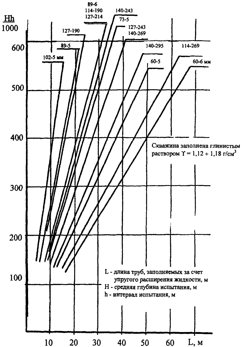
Рисунок 2.2.3 Определение упругого расширения пластовой жидкости
