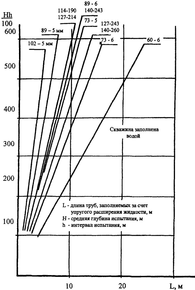
Рисунок 2.2.4 Определение упругого расширения пластовой жидкости
