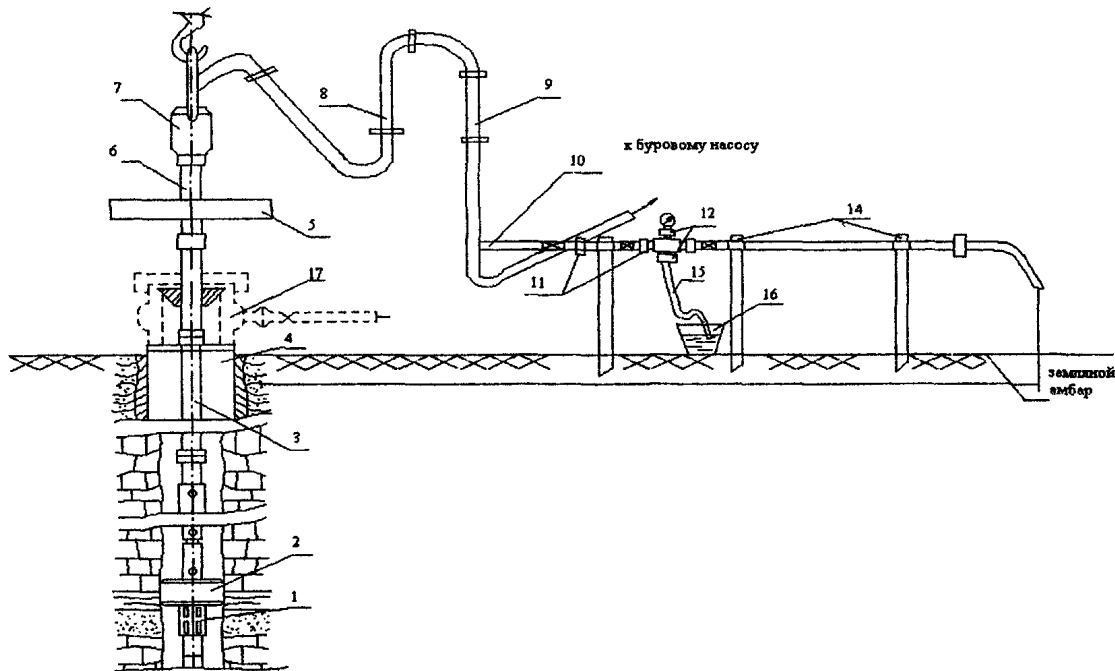
Рисунок 6. 3. 3. Схема обвязки устья скважины при испытании ИПТ:
