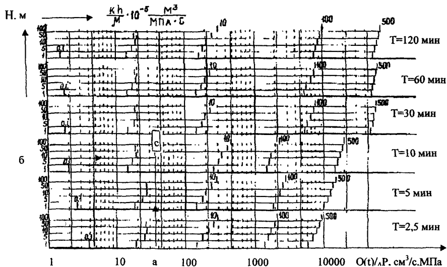
Рисунок 2.2.1 Определение гидропроводности призабойной зоны (испытание на бурильных трубах, d=114-127 \text{ мм} ). Шифр кривых: интервал испытания, Н, м. Исходные данные: Q(t)/\Delta P(t) , Т, Н. Порядок построения: абс
