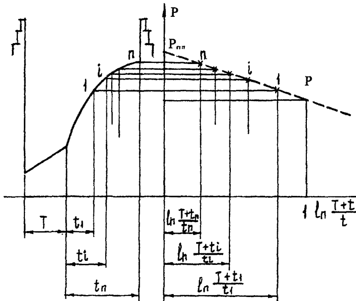
Рисунок 2.1.1 График Хорнера при обработке КВД:
