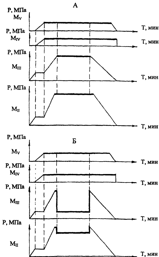
Рисунок 1.2.4 Диаграммы изменения забойного давления под фильтром ( M_{II} ), в фильтре ( M_{III} ), между КЦ и ЗП ( M_{IV} ) и в трубах над ИПТ ( M_V ) при закрытом впускном клапане и при полностью заглинизированных щелях фильтра.
