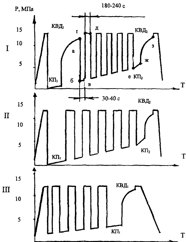
Диаграммы давления глубинного манометра ИПТГ в процессе исследования и очистки пласта гидроударами
