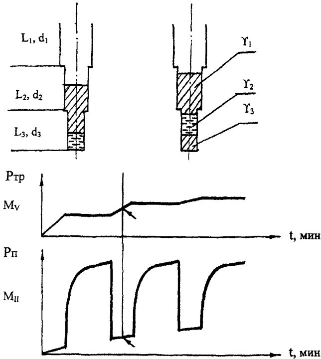
Рисунок 1.1.11 Схема притока в трехсекционную колонну бурильных труб и диаграммы давления на забое ( M_v ) и в трубах над ИПГ ( M_p ) при испытании пласта низкой гидропроводности
