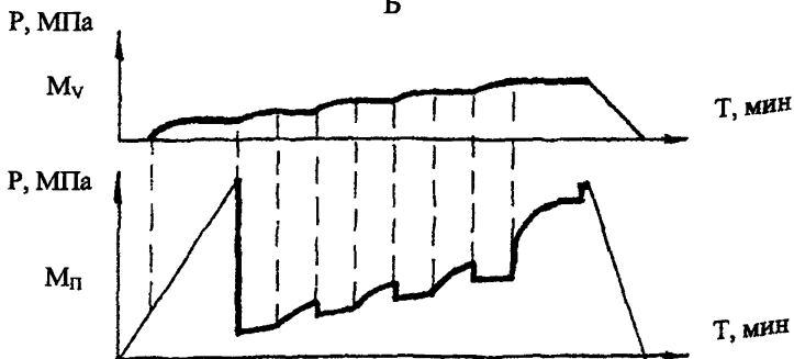
Рисунок 1.2.5 Диаграммы изменения давления под фильтром ( M_{II} ), в фильтре ( M_{ш} ), между КЦ и ЗП ( M_{IV} ) и в трубах над испытателем ( M_V ) при полном (А) и периодическом (Б) засорении фильтра.
