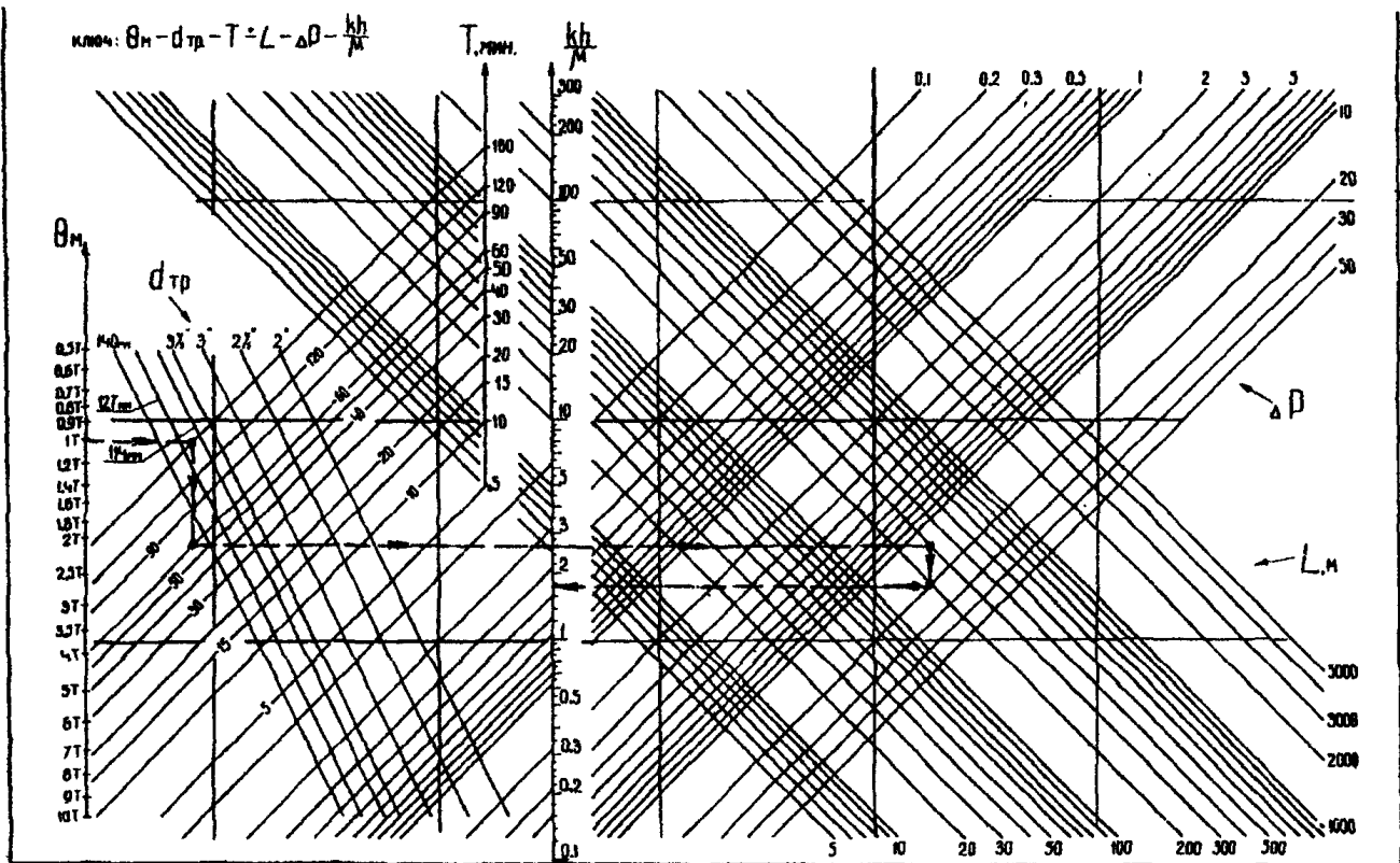
Рисунок 2.1.3 Номограмма для определения kh/\mu по КВД
