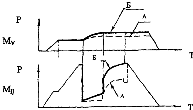
Рисунок 1.1.3 Диаграммы одноциклового испытания низкопроницаемого пласта:
