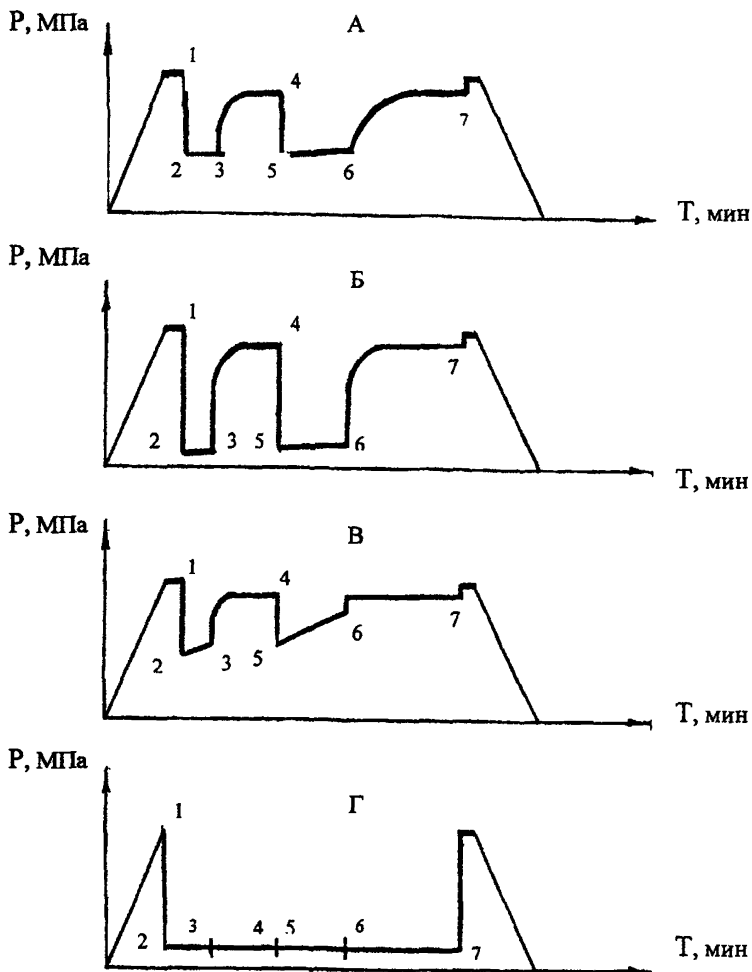
Рисунок 1.1.12 Диаграммы (основные типы) изменения забойного давления при испытании пластов ИПГ в обсадной колонне: А - проницаемый пласт; Б - проницаемый пласт с призабойной закупоркой; В - высокопроницаемый пласт; Г - «сухой» пласт.
