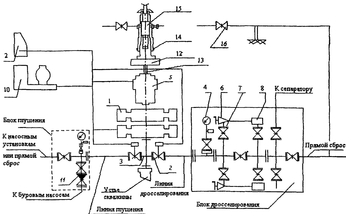
Рисунок 6.3.1 Схема обвязки устья скважины:
