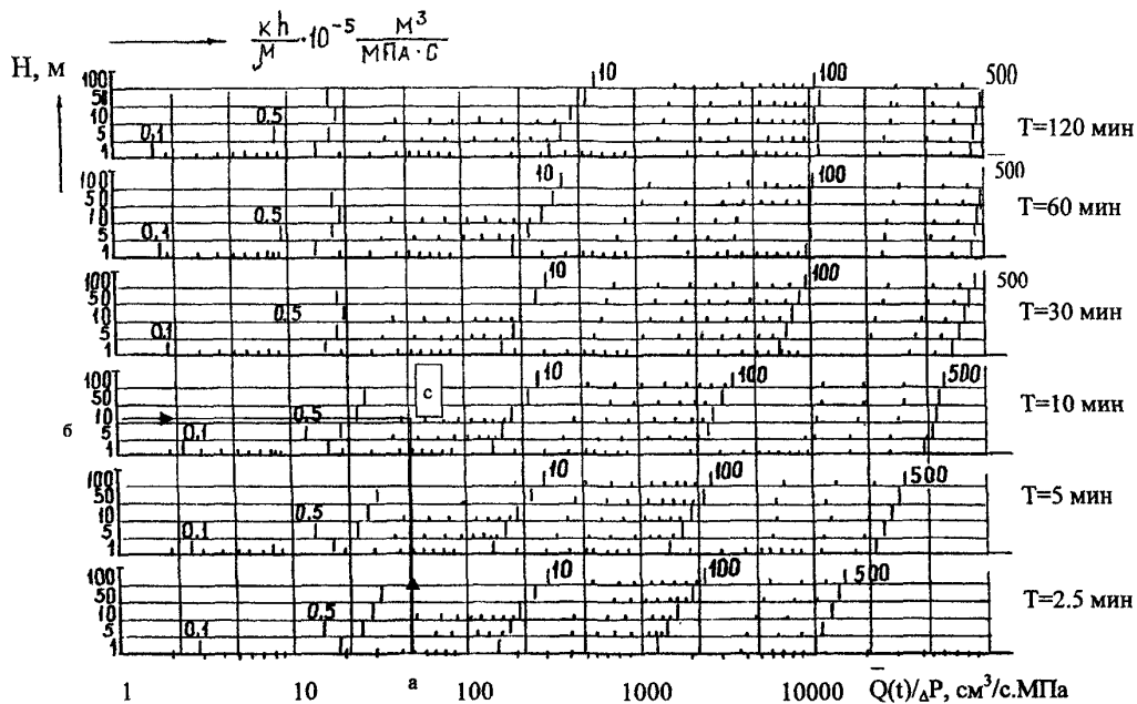
Рисунок 2.2.2 Определение гидропроводности призабойной зоны (испытание на НКТ)
