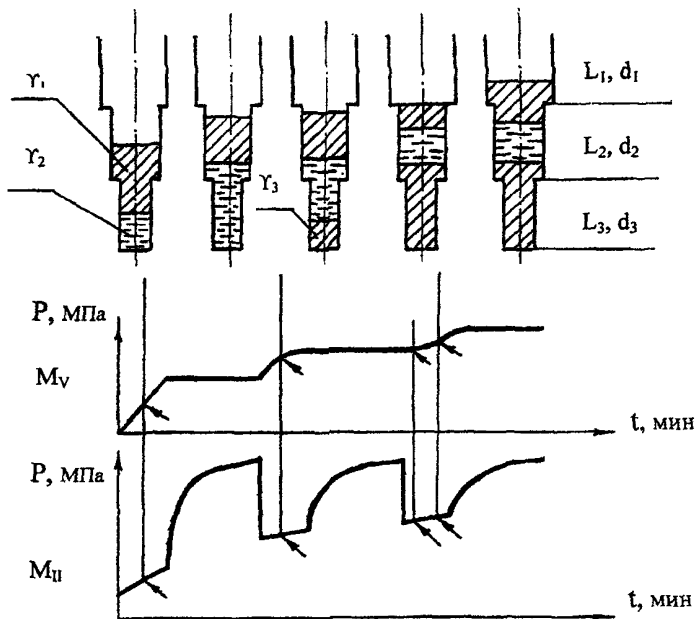
Рисунок 1.1.10 Схема притока в трехсекционную колонну бурительных труб и диаграммы давления на забое ( M_{ц} ) и в трубах над ИПТ ( M_{v} ) при испытании пласта высокой гидропроводности.
