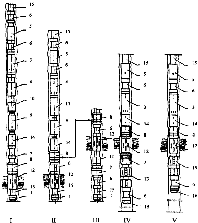
Типовые компоновки КИИЗ-146 с опорой (I, II, III) и без опоры (IV, V) на забой скважины:
