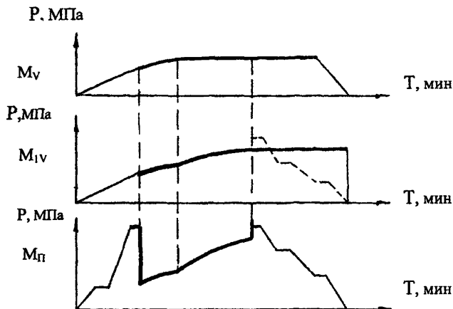
Рисунок 1.2.6 Диаграммы изменения давления на забое ( M_{п} ), между КЦ и ЗП ( M_{IV} ) и в трубах ( M_v ) при негерметичном клапане ИПТ
