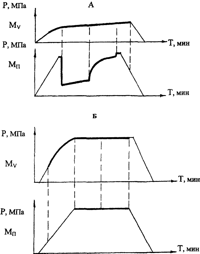
Рисунок 1.2.2 Диаграммы изменения давления, записанные манометром M_v в трубах и M_{п} на забое при частичной (А) и полной негерметичности (Б) труб над ИПТ
