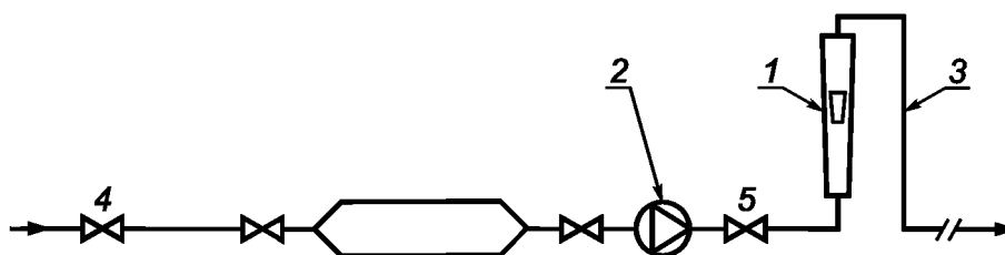
1 — ротаметр; 2 — диафрагменный насос (взрывобезопасный); 3 — линия сброса; 4 — точка отбора пробы; 5 — клапан ротаметра
