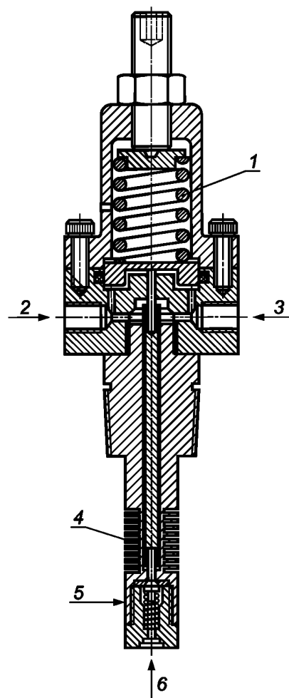
1 — пружина, регулирующая выход; 2 — к манометру и сбросу; 3 — выход газа; 4 — тепловые ребра; 5 — точка регулировки; 6 — вход газа
