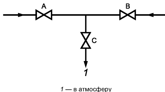
Рисунок А.1 — Принцип двойной блокировки и сброса
