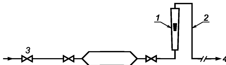
1 — ротаметр; 2 — линия сброса; 3 — точка отбора пробы; 4 — раструб или сброс
