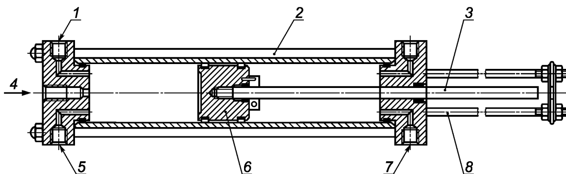
1 — отверстие сброса; 2 — стяжные болты; 3 — индикаторный стержень; 4 — пробка; 5 — отверстие для манометра и клапана; 6 — поршень; 7 — предварительная заправка; 8 — штатив-ограничитель (стержень поршня выдвигается на 80 %)
