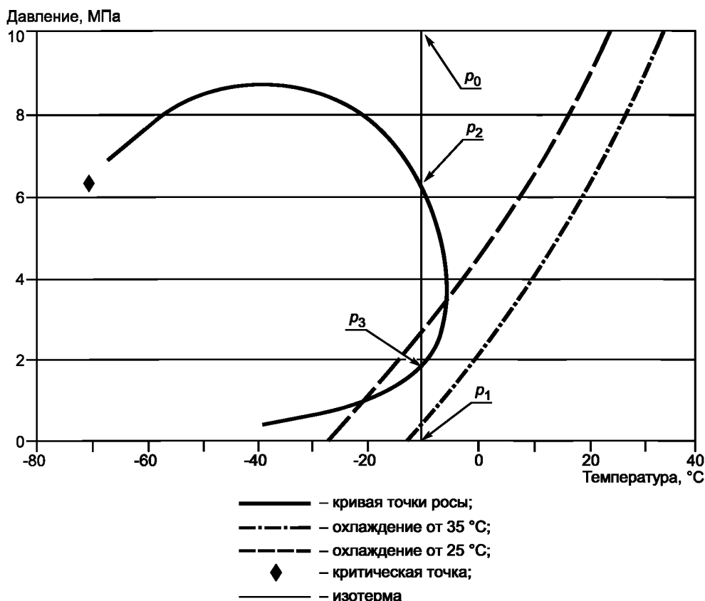
Рисунок 2 — Пример диаграммы давление/температура для природного газа
