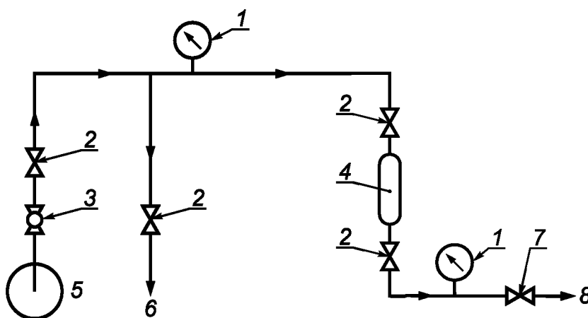
1 — манометр; 2 — вентиль; 3 — шаровой вентиль; 4 — контейнер для пробы; 5 — зонд; 6 — сброс; 7 — выходной вентиль; 8 — трубка, идущая к измерителю скорости потока — трубе Вентури
