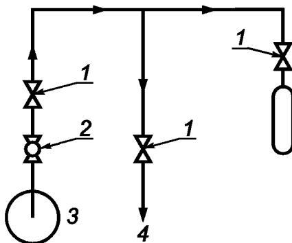
1 — вентиль; 2 — шаровой вентиль; 3 — зонд; 4 — сброс
