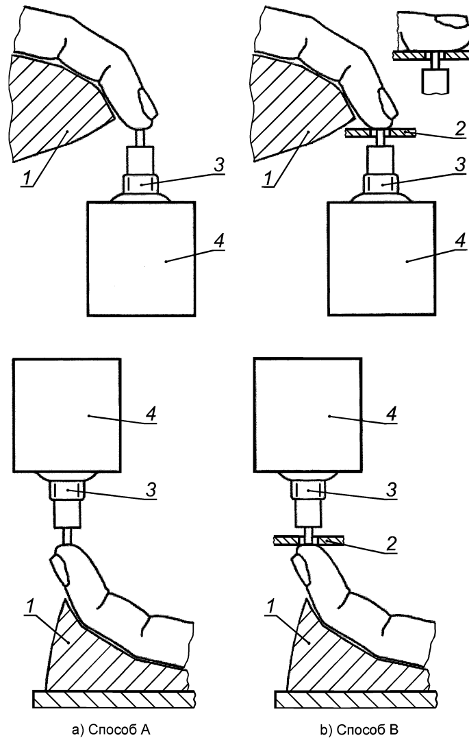
Рисунок 1 — Способы опирания пальца, на который воздействует толкатель
