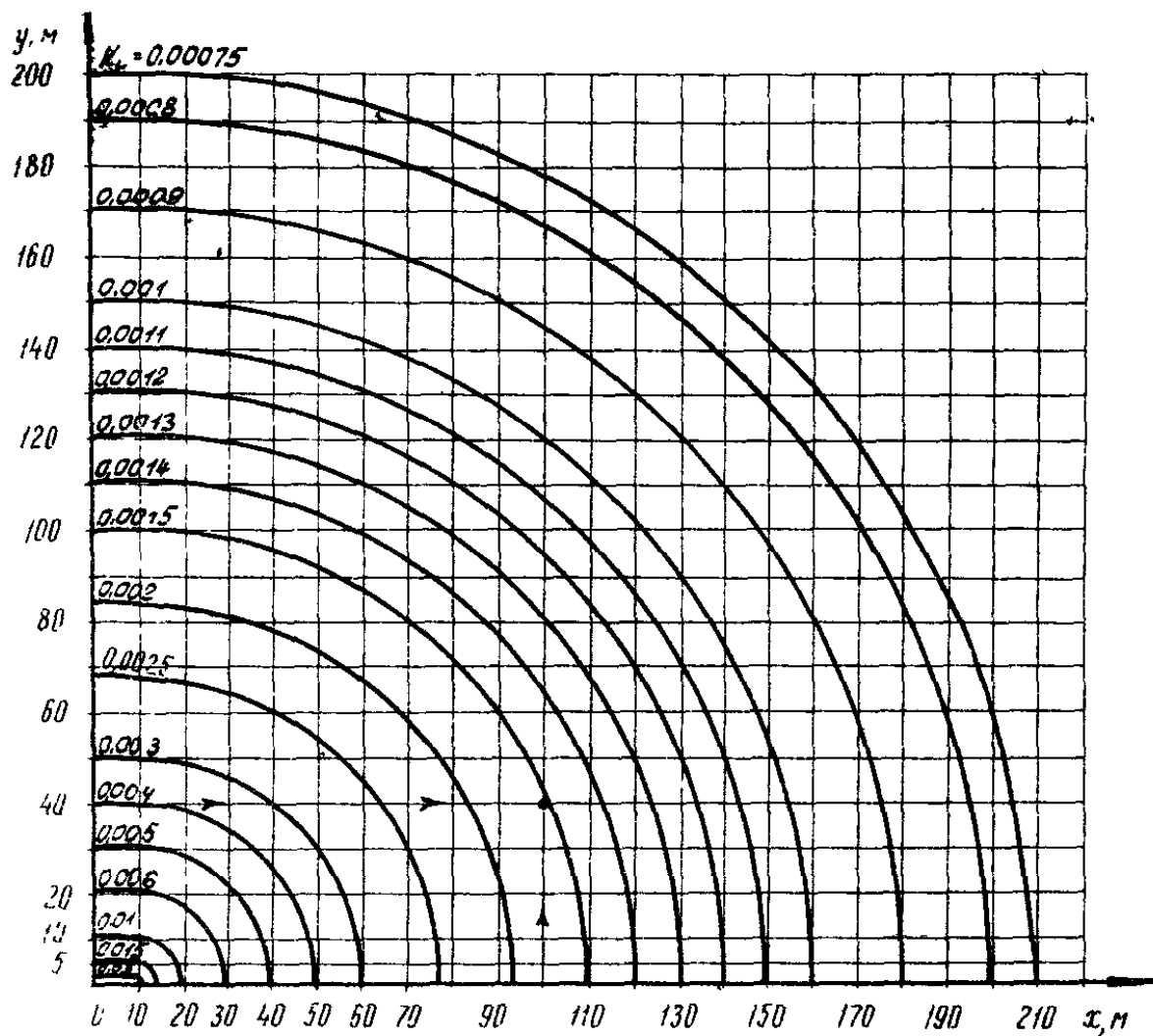
Рис.14. Коммуникация длиной 20 м
