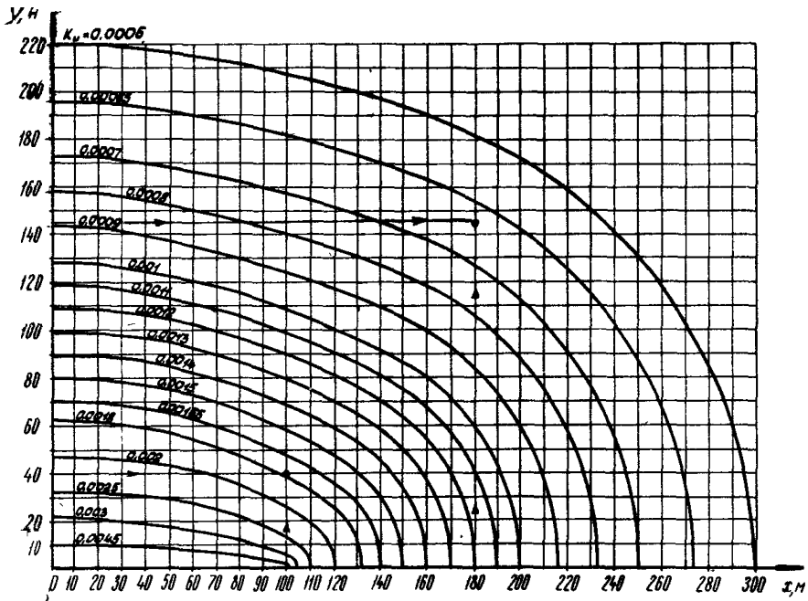
Рис.27. Коммуникация длиной 200 м
