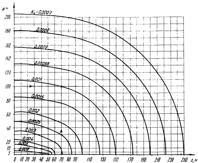
Рис.22. Коммуникация длиной 100 м
