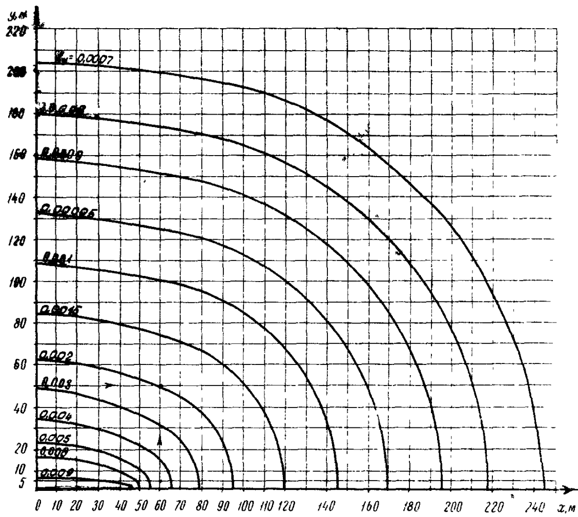
Рис.21. Коммуникация длиной 90 м
