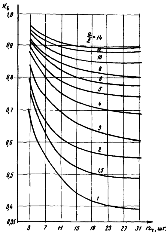
Рис.6. Зависимость коэффициента экранирования вертикальных заземлителей в коксовом активаторе K_6 от числа электродов n_3 при различных отношениях \frac{a}{2} :
