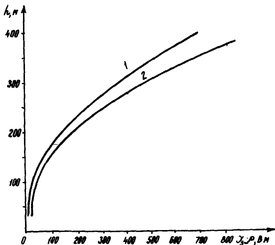
Рис.10. Зависимость глубины заложения анодного заземления h от напряженности поля у анодного заземления U_3, \rho для площадки 250 \times 180 м:
