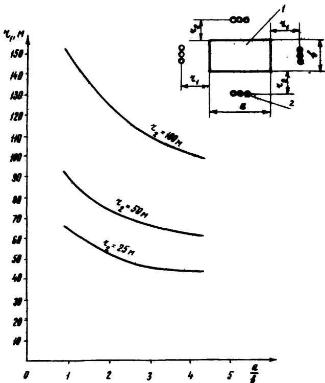
Рис.5. Зависимость величины отброса сосредоточенных анодных заземлений от соотношения сторон площадки:
