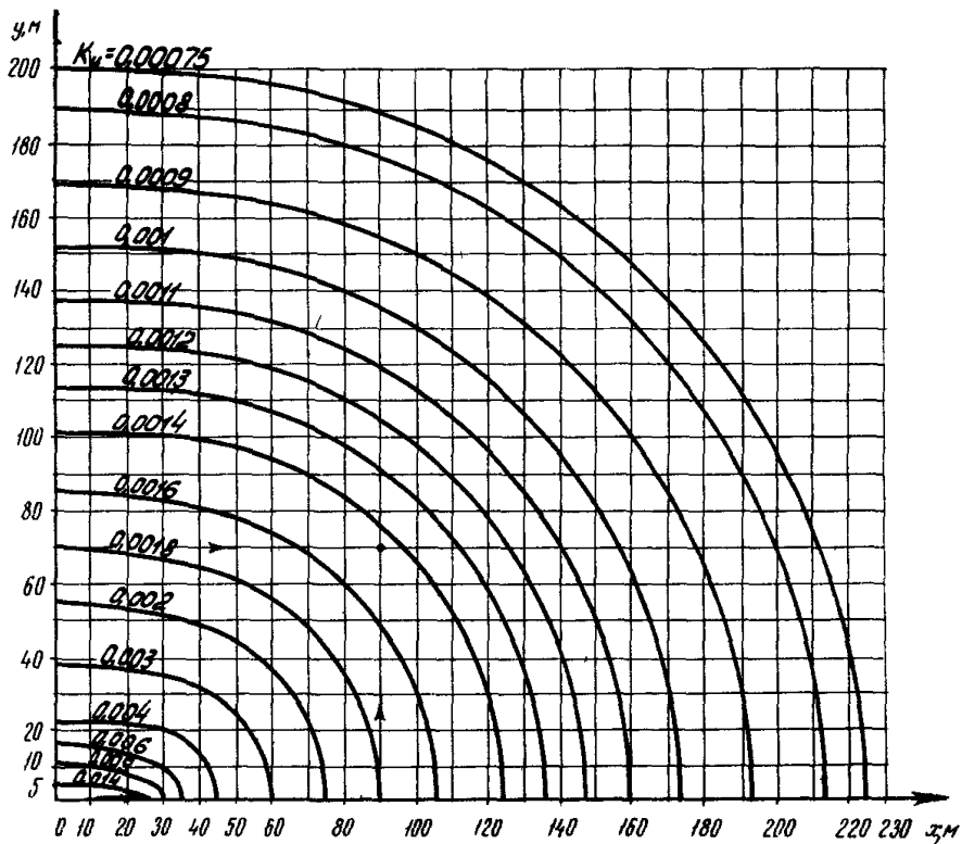
Рис. I7. Коммуникация длиной 50 м
