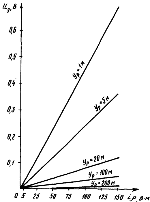
Рис.3. Зависимость потенциала земли U_3 от напряженности поля E_p сооружения длиной 20 м в точке, удаленной от сооружения на расстояниях r_p
