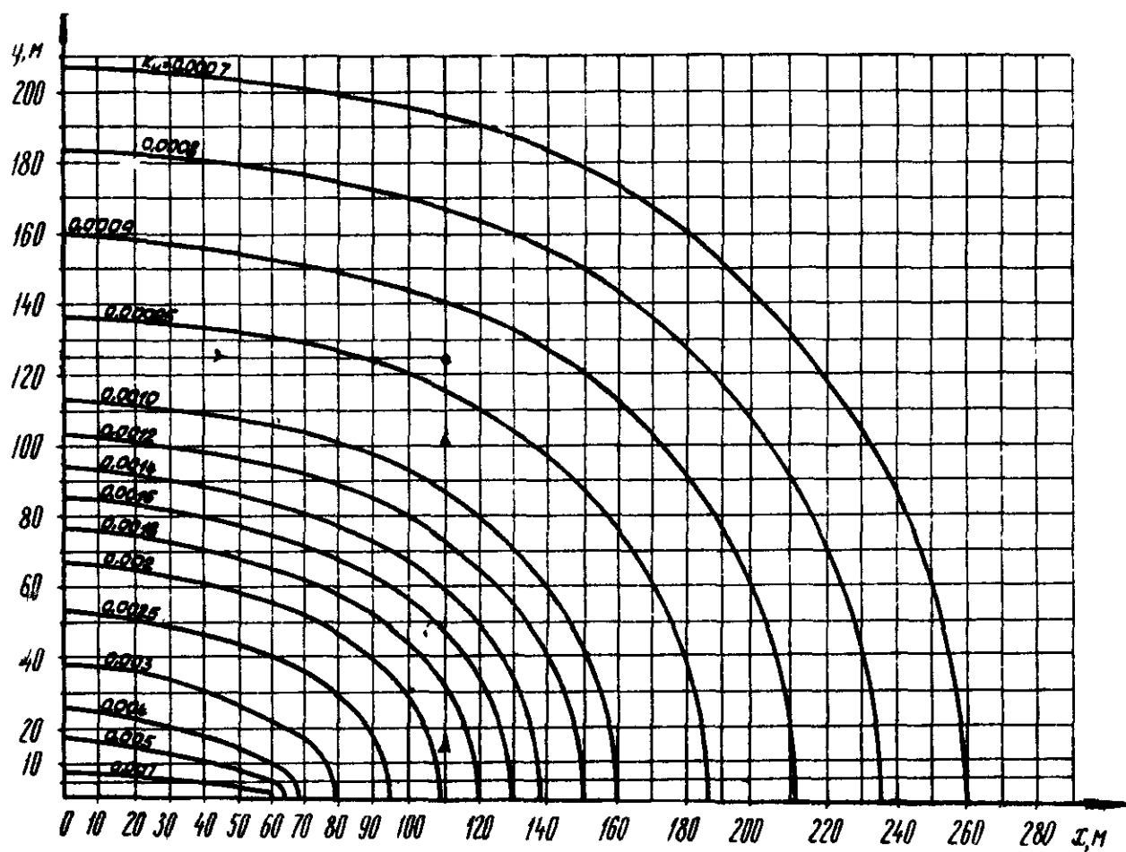
Рис.23. Коммуникация длиной 120 м
