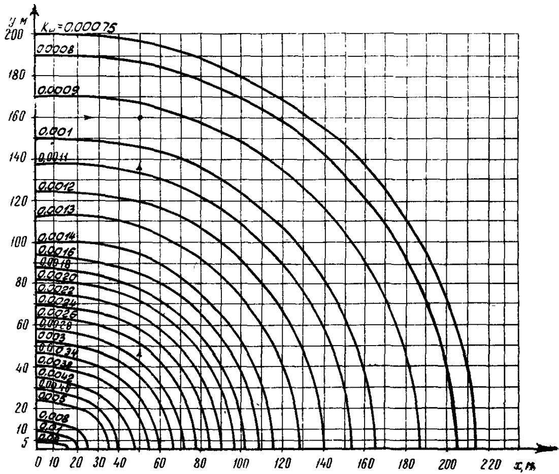
Рис.15. Коммуникация длиной 30 м
