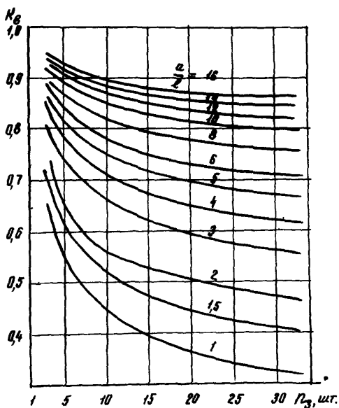
Рис.9. Зависимость коэффициента экранирования горизонтальных заземлителей K_g от числа электродов n_3 при различных отношениях \frac{a}{l} : a - расстояние между заземлителями, м; l - длина заземлителей 3 м, глубина установки 1,5 м
