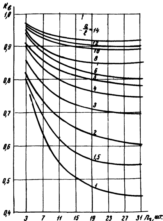
Рис.8. Зависимость коэффициента экранирования горизонтальных заземлителей в коковом активаторе K_B от числа электродов n_3 при различных отношениях \frac{a}{l} . a —расстояние между заземлителями, м; l —длина заземлителей 1,4 м, глубина установки 1,7 м
