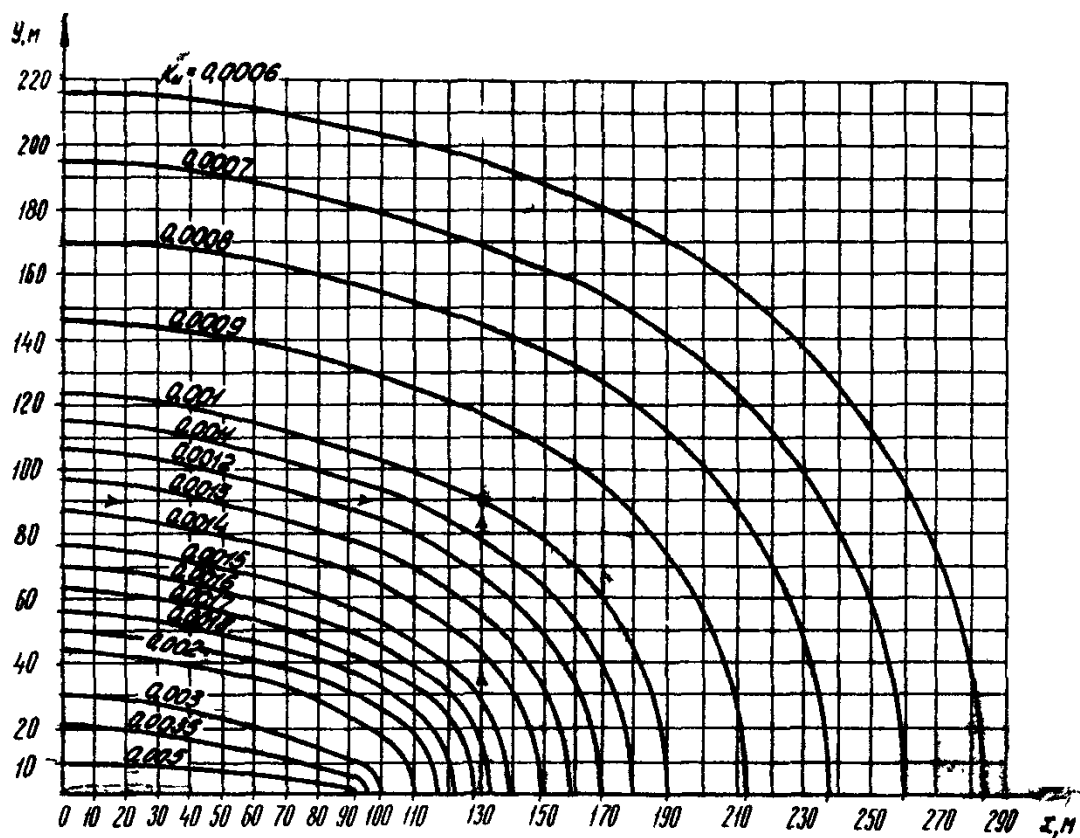
Рис.26. Коммуникация диной 180 м
