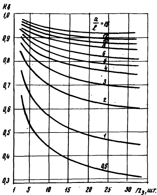
Рис.7. Зависимость коэффициента экранирования вертикальных заземлителей K_\phi от числа электродов n_3 при различных отношениях \frac{a}{l} : a — расстояние между заземлителями, м; l — длина заземлителей 3 м, глубина установки 3 м
