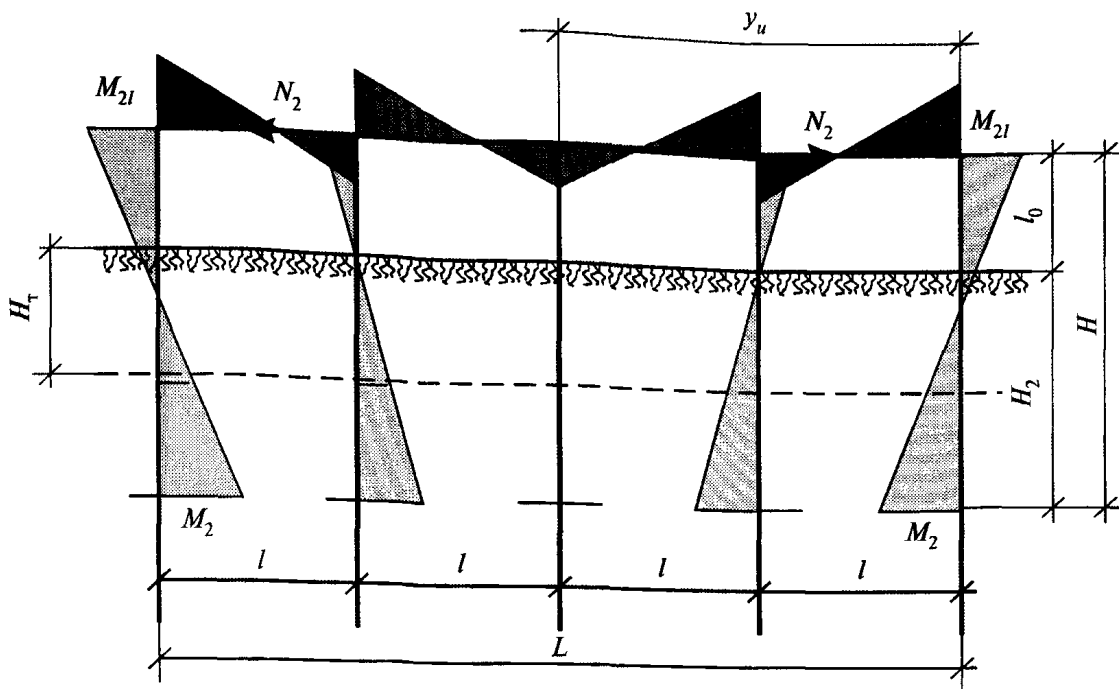
a — первая стадия работы при замороженном грунте — зимой; б — вторая стадия работы при оттаявшем грунте — летом Рисунок 7.2 — Эпюры моментов в свайном фундаменте с жесткой заделкой свай в фундаментную балку от воздействия температуры и влажности воздуха
