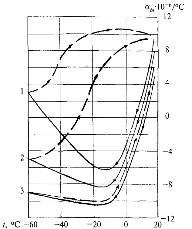
— при замораживании; - - - при оттаивании; 1, 2, 3 — условия работы конструкции по табл. 4.1
