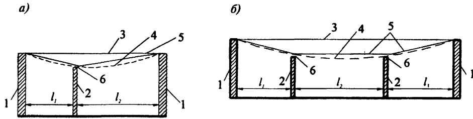
Рисунок Г.1 — Схемы для определения значений l ( l_1, l_2, l_3 ) при наличии между стенами капитальных перегородок a — одной в пролете; b — двух в пролете; 1 — несущие стены (или колонны); 2 — капитальные перегородки; 3 — перекрытие (покрытие) до приложения нагрузки; 4 — перекрытие (покрытие) после приложения нагрузки; 5 — линии отсчета прогибов; 6 — зазор
