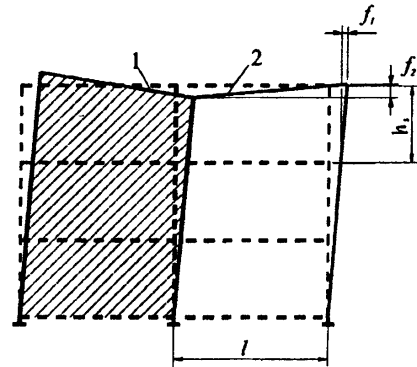
Рисунок Г.3 — Схема перекоса этажных ячеек 2, примыкающих к диафрагмам жесткости 1 в зданиях со связевым каркасом (пунктиром показана исходная схема каркаса до приложения нагрузки)
