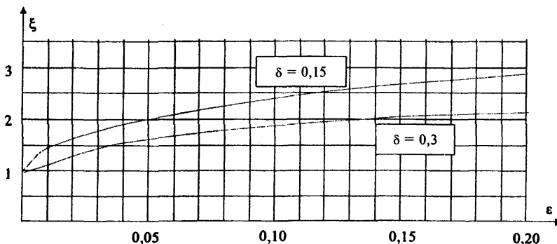
Рисунок 6.1 — Коэффициенты динамичности
