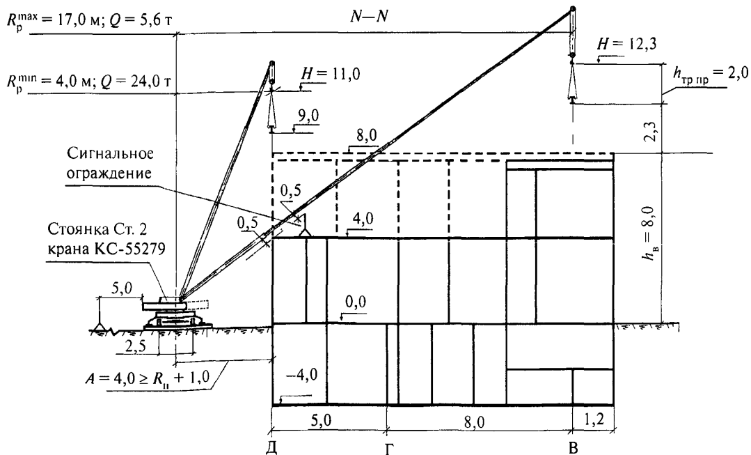
Рисунок 2. Вертикальная привязка монтажного крана
