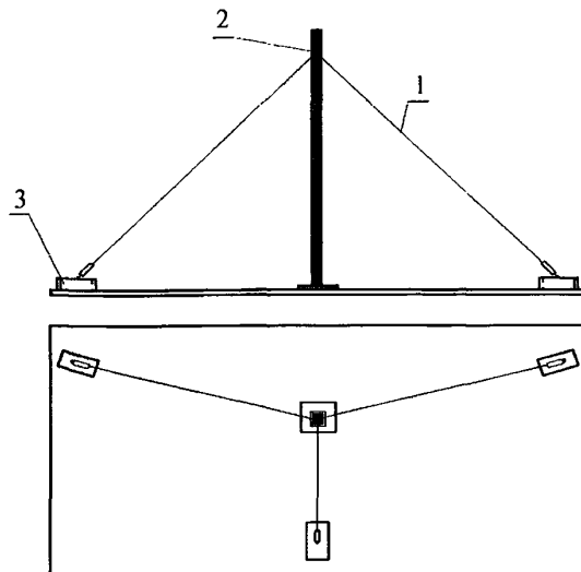
Рисунок 4. Временное закрепление колонны
