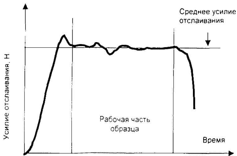
Рисунок 4 - Типичная кривая при проведении испытаний на адгезию
