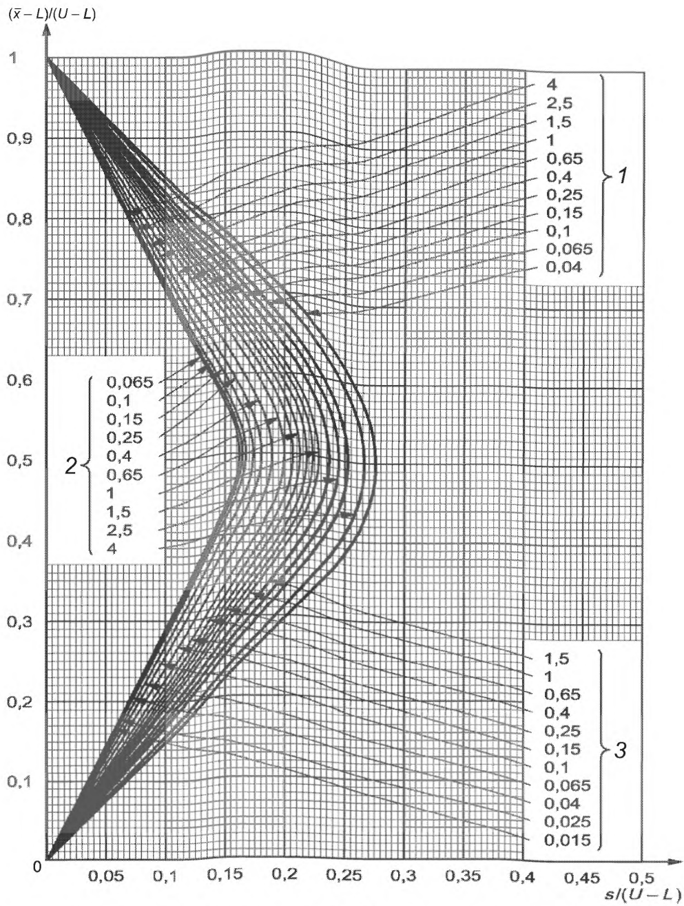
Рисунок 28 — График s-M. Приемочные кривые для объединенного контроля с двумя пределами поля допуска и общим AQL. «s» метод. Код объема выборки M (объем выборки 95) (для ослабленного контроля код объема выборки P)
