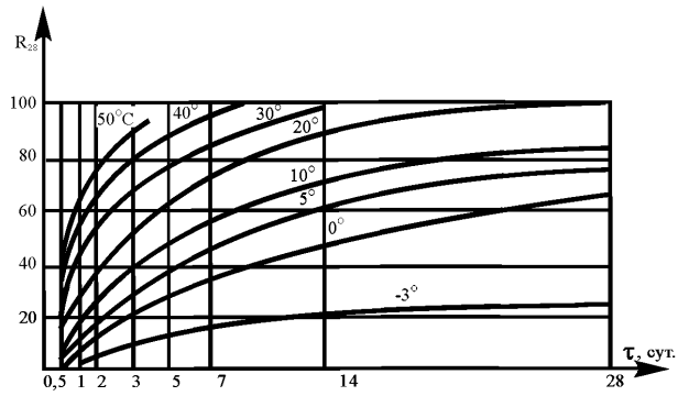
Рисунок 2 – График нарастания прочности бетона класса В15, В25 на портландцементе марки 400
