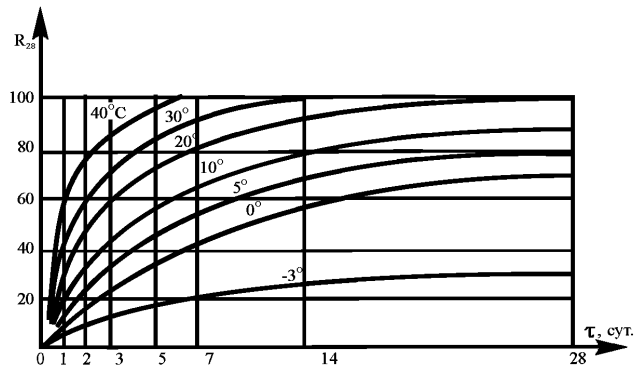
Рисунок 3 – График нарастания прочности бетона класса В35 на портландцементе марки 500
