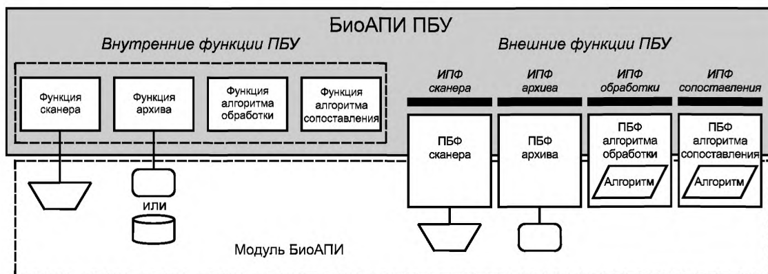
Рисунок 2 — Иллюстрация архитектуры ПБУ
