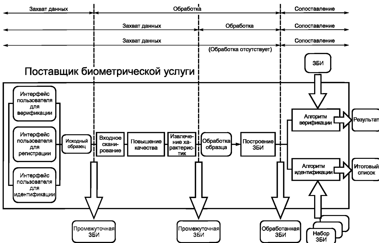
Рисунок С.1 — Возможная архитектура реализации технологии БиоАПИ
