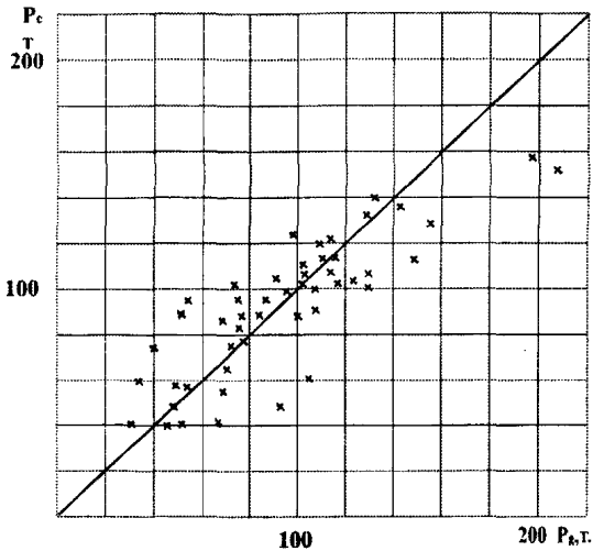
Рис.18. График сравнения допустимо-предельной нагрузки на сваю по статическим испытаниям P_c и определенной по сопротивлению погружению P_q .
