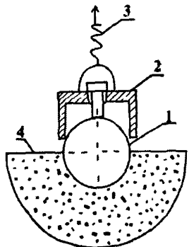
Рис 15 Глиномер ГЕ-6. Основные части: 1 – шар, 2 – обойма, 3 – динамометр, 4 – грунт. Габаритные размеры в упаковке 4,5x10x15 см, вес 0,4 кг. Служит для установления типа глинистого грунта с подразделением на глинистый песок, супесь, суглинок, глину. Время испытания 5-10 минут, без сушки и взвешивания. Одновременно может использоваться для определения липкости.
