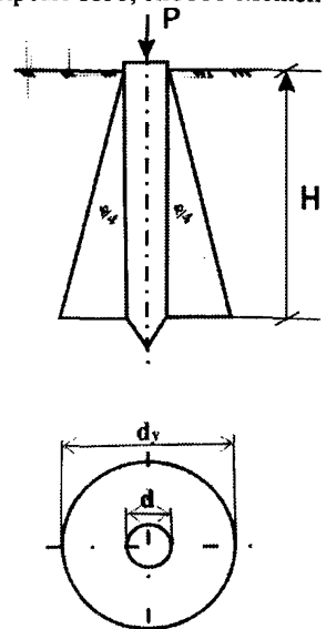
Рис. 19. Схема определения площади условного фундамента под свайей.
