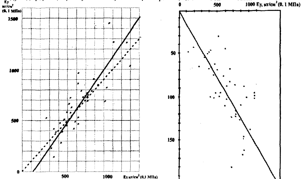
Рис. 20. Графическое сопоставление модулей деформации верхнепермских глин, определенных по результатам статических испытаний свай E_y по (43) и сопротивлению погружению конуса E_3 по (19): сплошная линия – аппроксимирующее значение; пунктир – среднее значение.
