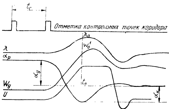
Образец записи параметров при испытаниях «поворот R_{II} = 25 м»
