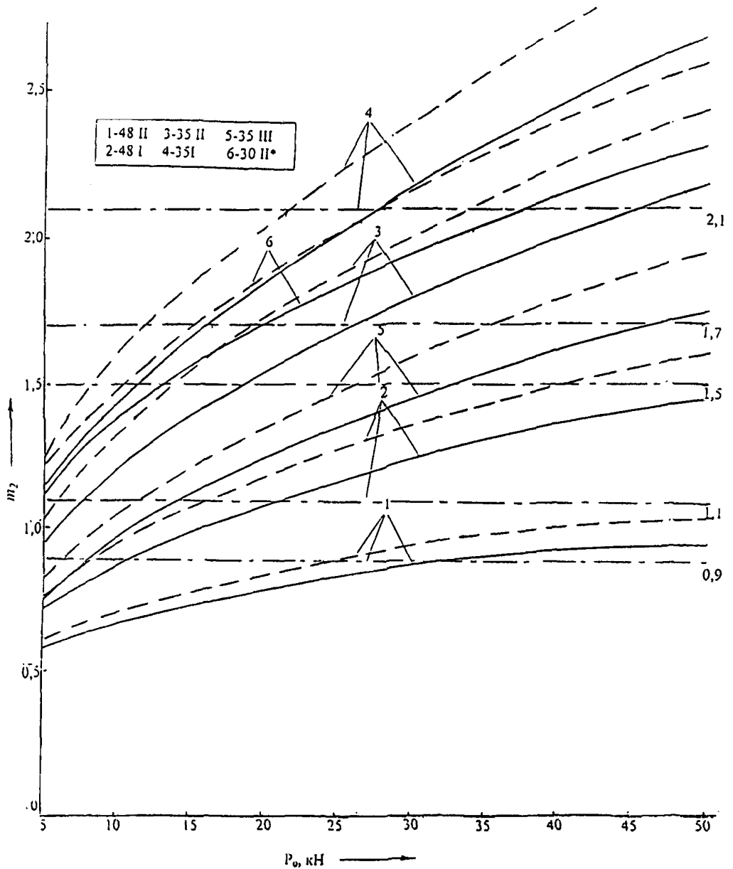
Рис. 4. Зависимости m_2 от P_0 и типа анкера по ГОСТ 22690 истоящей методике заполнители: • — гранитный • - - - мелкозернистый или гравийный
