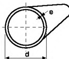
Размеры труб ИКАПЛАСТ из полиэтилена для газопроводов по ГОСТ Р 50838-95 и ТУ 2248-002-50049230-2004
