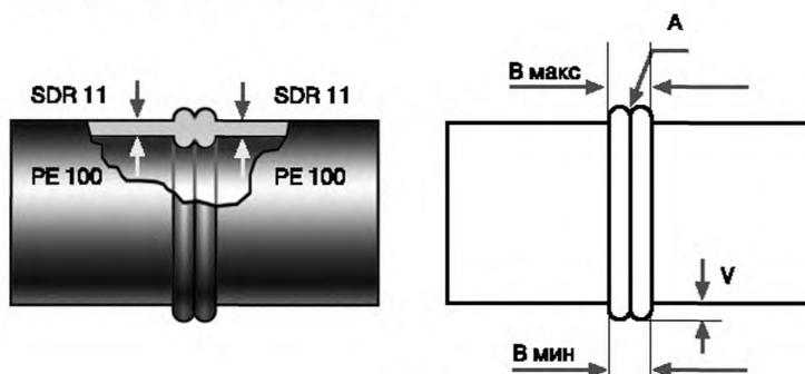
Рис 4.2.19 Параметры грата
