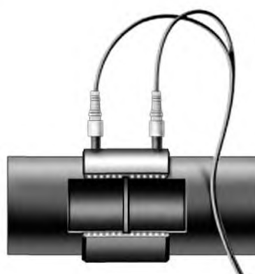
Рис 4.2.2 Соединение труб муфтой с ЗН
