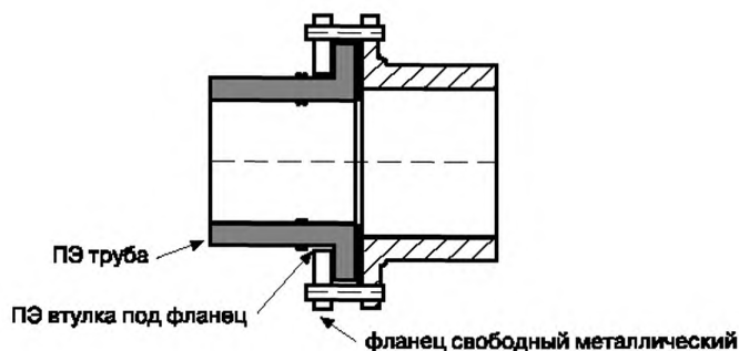
Рис. 1.1 Схема фланцевого соединения
