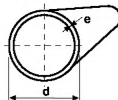
Сортамент труб ИКАПЛАСТ из полиэтилена по ГОСТ 18599-2001
