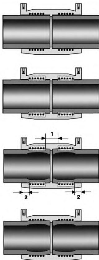
Рис 4.2.5 Процесс сварки муфтой с ЗН
